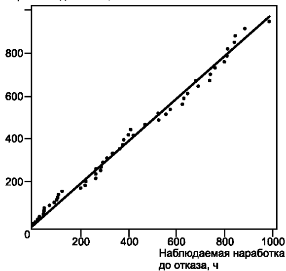
Математическое ожидание наработки до отказа, ч
