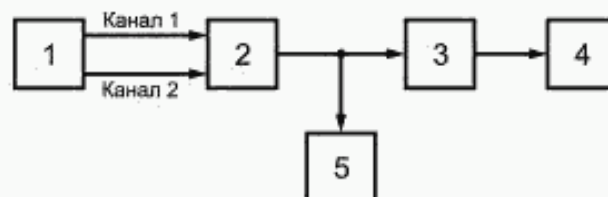
Рисунок 20 — Схема измерения краевых искажений телеграфных сигналов
