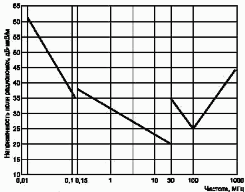
Рисунок 3 — Нормы напряженности поля радиопомех
