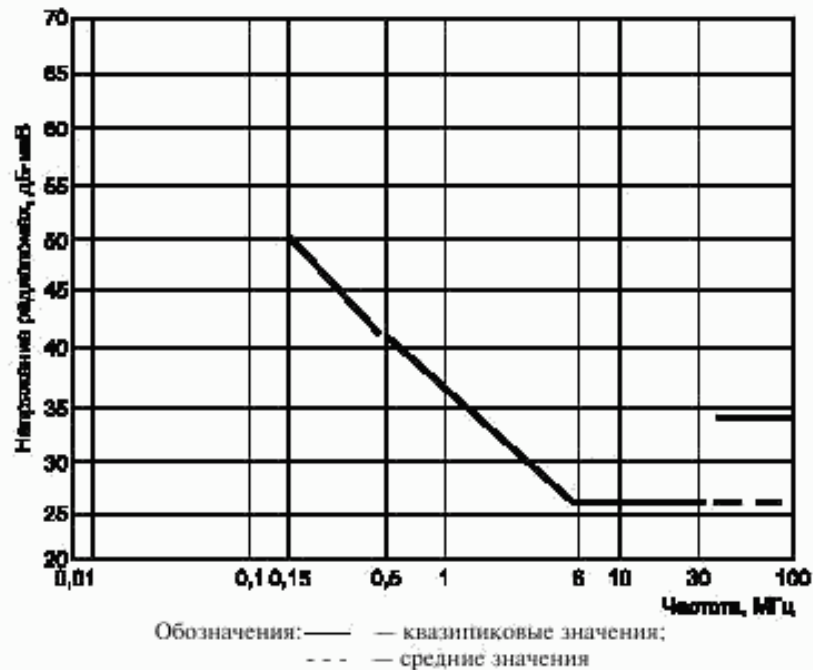
Рисунок 2 — Нормы напряжения радиопомех
