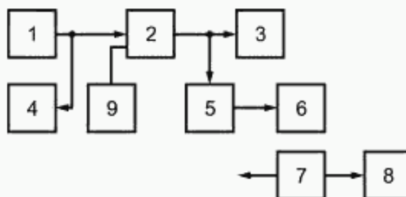
Рисунок 10 — Схема измерения уровня линейных переходных искажений между однополосными каналами
