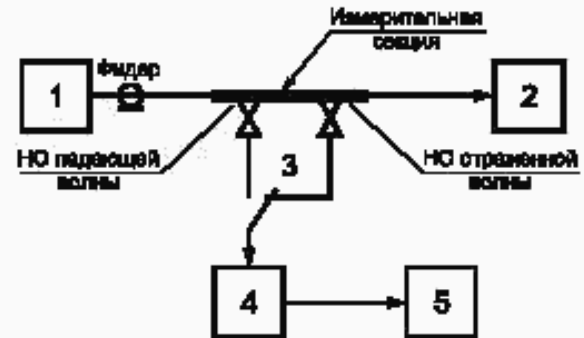
Рисунок 26 — Схема измерения средней мощности побочных радиоколечаний
