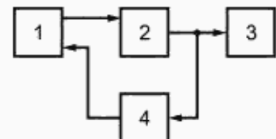
Рисунок 14 — Схема измерения неравномерности характеристики ГВЗ телефонных каналов
