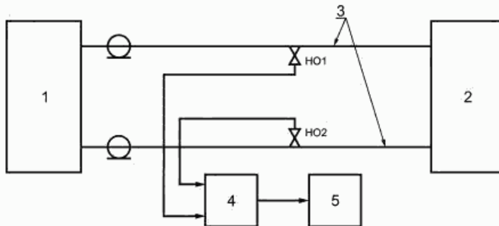
Рисунок Д.3 — Устройство сумматора противофазных сигналов
