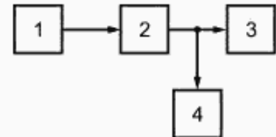
Рисунок 13 — Схема измерения среднего квадратического относительного уровня гармоник
