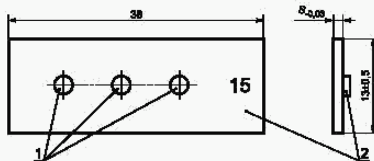
1 — отверстие \varnothing 1,6 мм; 2 — шифр пенетрометра
