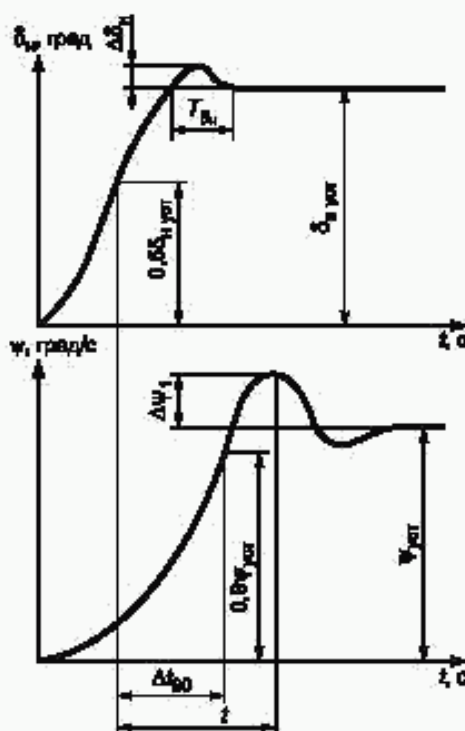
Рисунок 4 — Записи угла поворота рулевого колеса \delta_{в} и угловой скорости \psi автомобиля при испытании «рывок руля»
