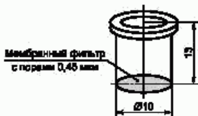
Рисунок 1 — Люминометрическая полистирольная кювета
