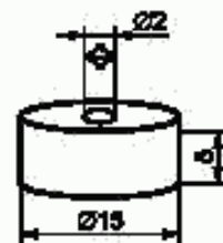
Рисунок 3 — Резиновый наконечник к медицинскому шприцу
