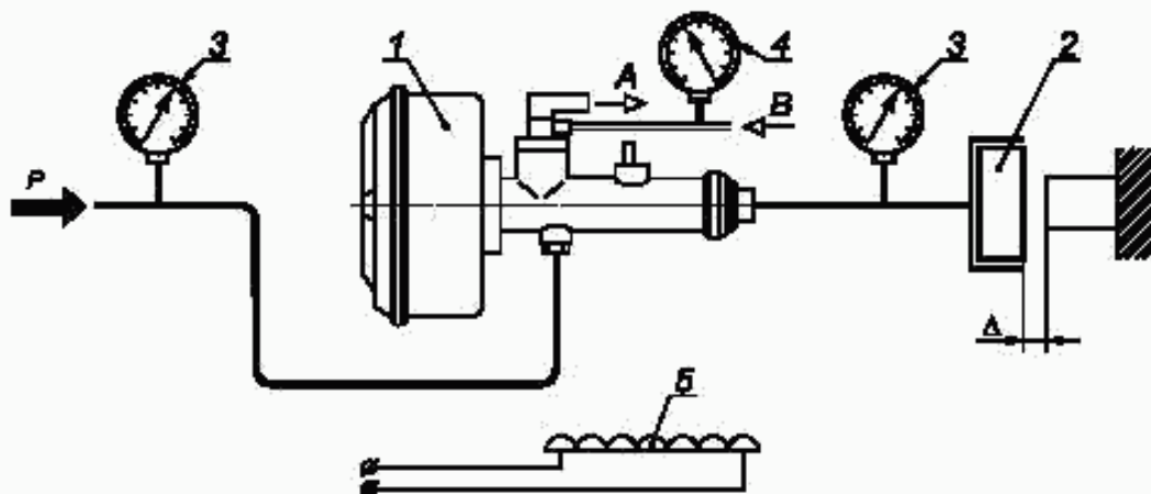
1 — объект испытаний; 2 — нагрузочный цилиндр; 3 — манометры; 4 — вакуумметр; 5 — нагревательный элемент; А — атмосфера; В — вакуум; P — давление на входе; Δ — зазор между штоком нагрузочного цилиндра и упором
