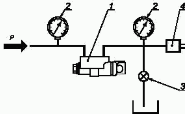
1 — объект испытаний; 2 — контрольные манометры; 3 — сливной храник; 4 — клапан прокачки; P — давление на входе Рисунок А.1 — Схема испытательной установки для определения функциональных свойств регуляторов тормозных сил гидравлического привода
