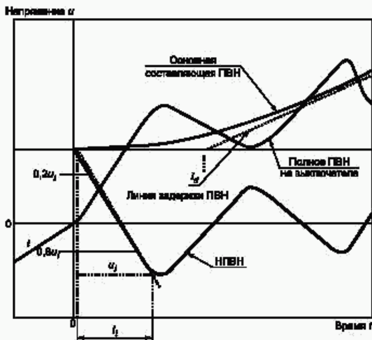
Рисунок 6 — Начальная часть переходного восстанавливающегося напряжения (НПВН)
