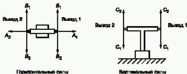
а) Статические нагрузки на выключатель
