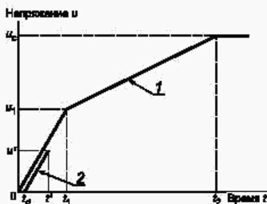
Рисунок 5 — Нормированные характеристики ПВН, определяемого четырьмя параметрами
