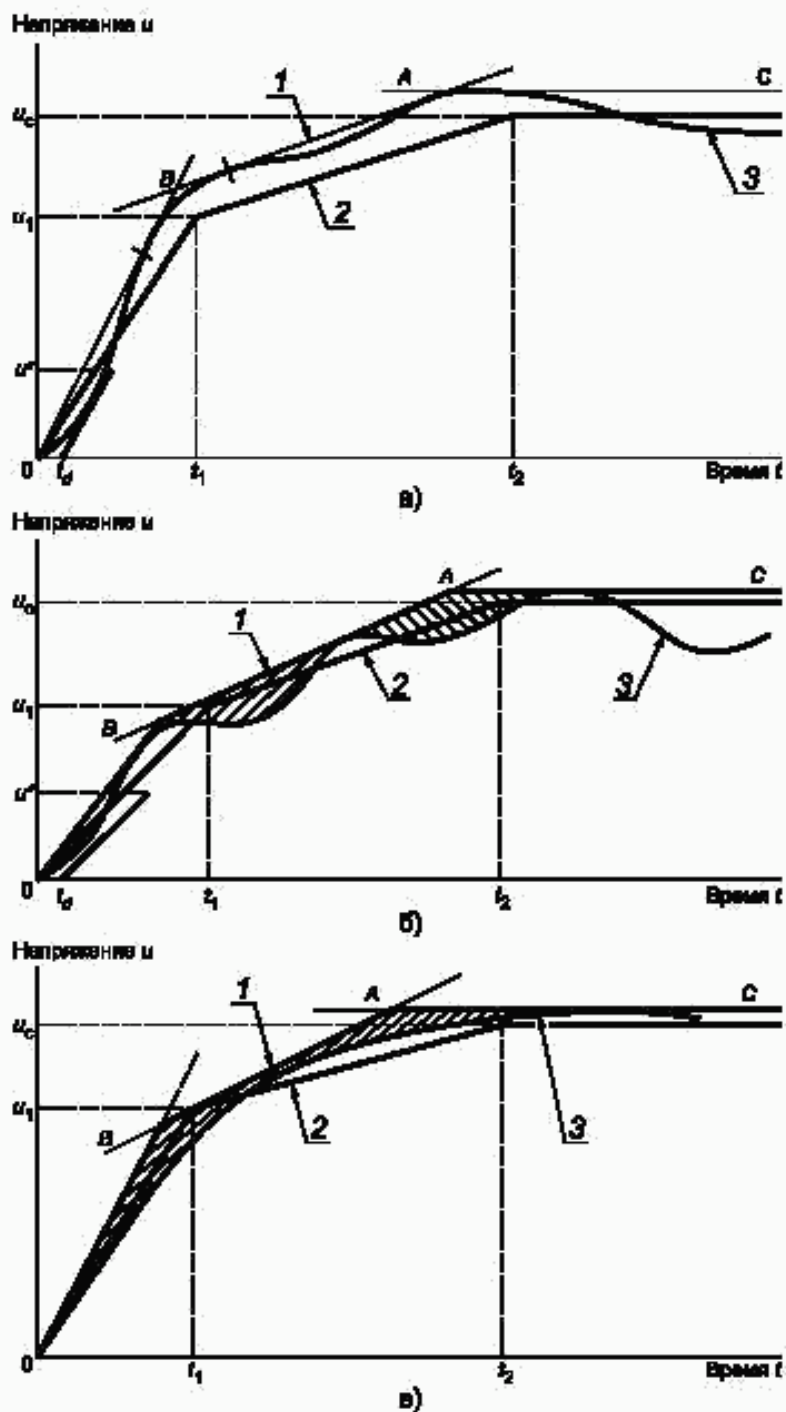
Рисунок В — Построение огибающей ПВН, определяемого четырьмя параметрами
