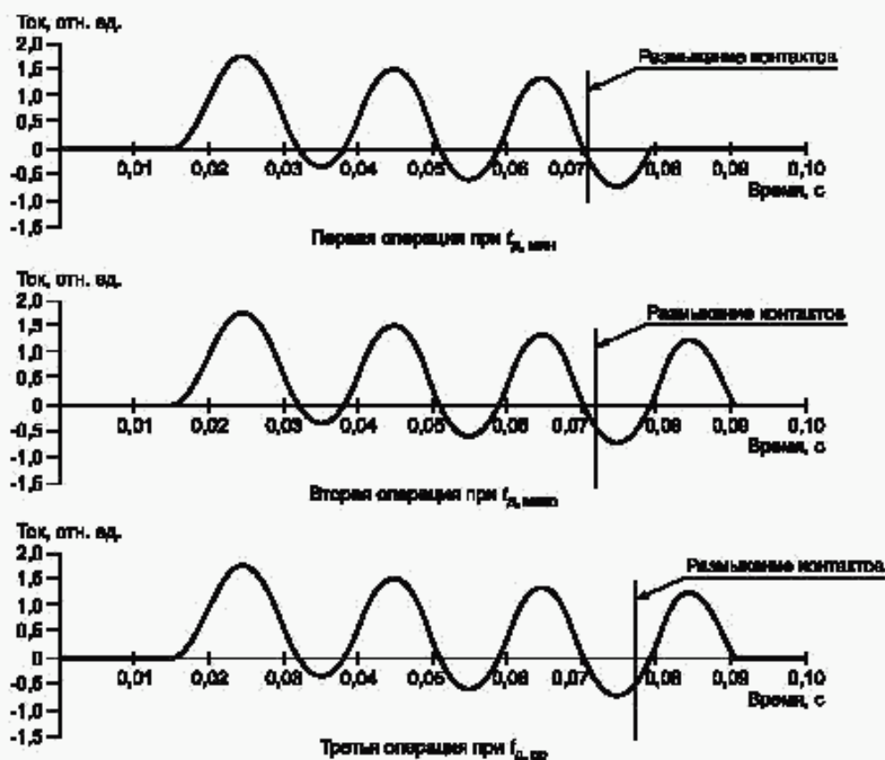
Рисунок 14 — Регулирование моментов инициирования тока и размыкания контактов при однополюсном отключении тока в режиме T100a выключателями с U_{ном} \geq 110 кВ
