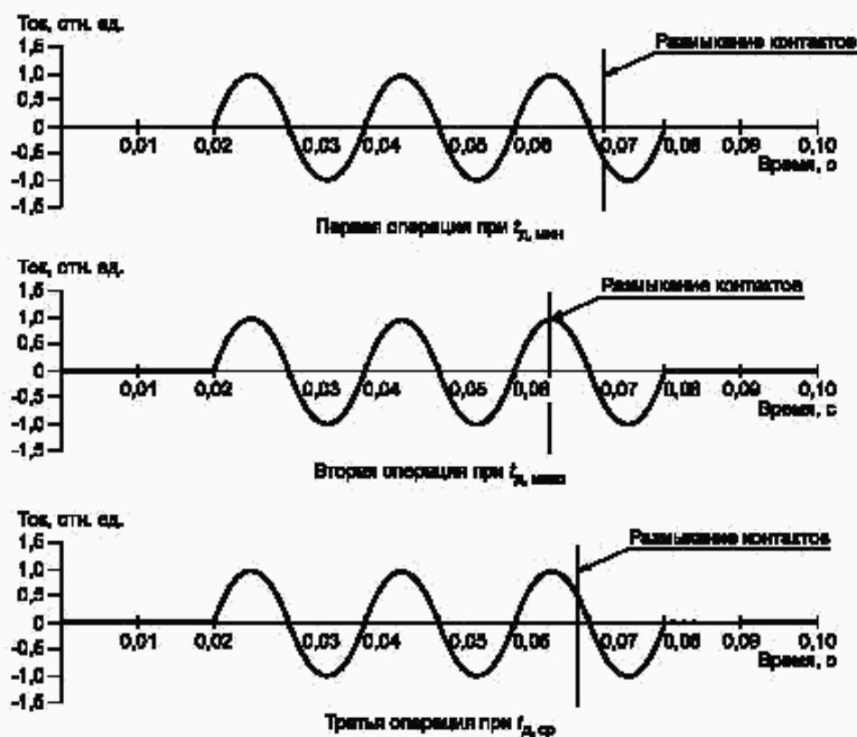
Рисунок 11 — Регулирование момента размыкания контактов относительно фазы тока при однополюсном отключении симметричного тока в режимах Т10, Т30, Т60, Т100с, Тсr1, Тсr2, Тсr3 выключателями с U_{ном} \leq 35 кВ
