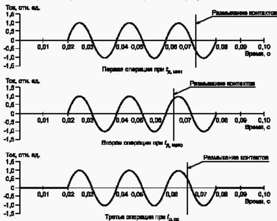
Рисунок 13 — Регулирование момента размыкания контактов относительно фазы тока при однополюсном отключении симметричного тока в режимах Т10, Т30, Т60, Т100S, Тcr1, Тcr2, Тcr3, OP2, L90, L75, L60 выключателями с U_{ном} \geq 110 кВ
