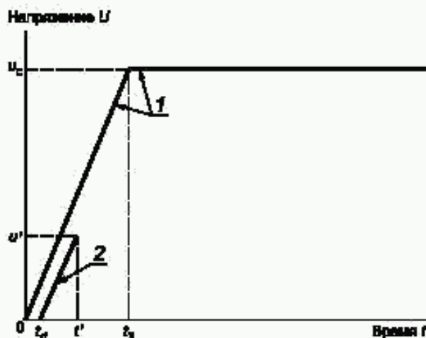
Рисунок 4 — Нормированные характеристики ПВН, определяемого двумя параметрами
