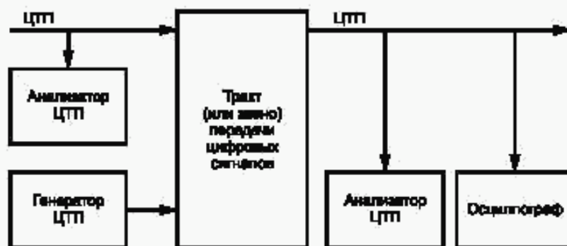
Рисунок 5.1 — Схема проведения измерений параметров цифрового транспортного потока
