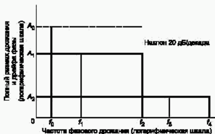
Рисунок 4.6 — Шаблон максимально допустимого входного фазового дрожания и дрейфа фазы
