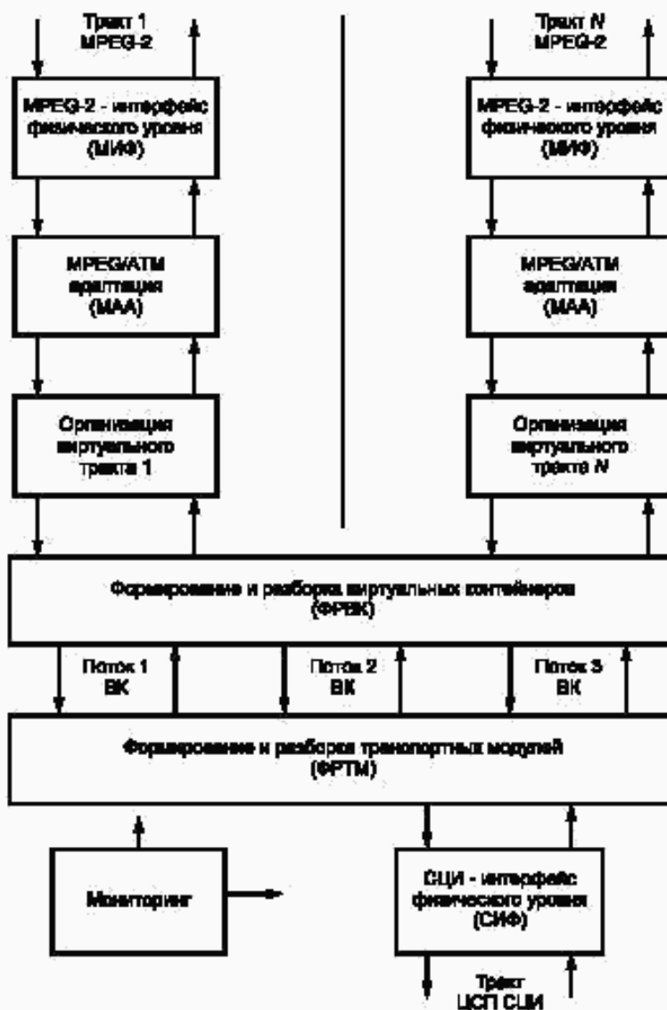
Рисунок 4.2 — Функциональная архитектура аппаратуры преобразования MPEG → СД и СД → MPEG
