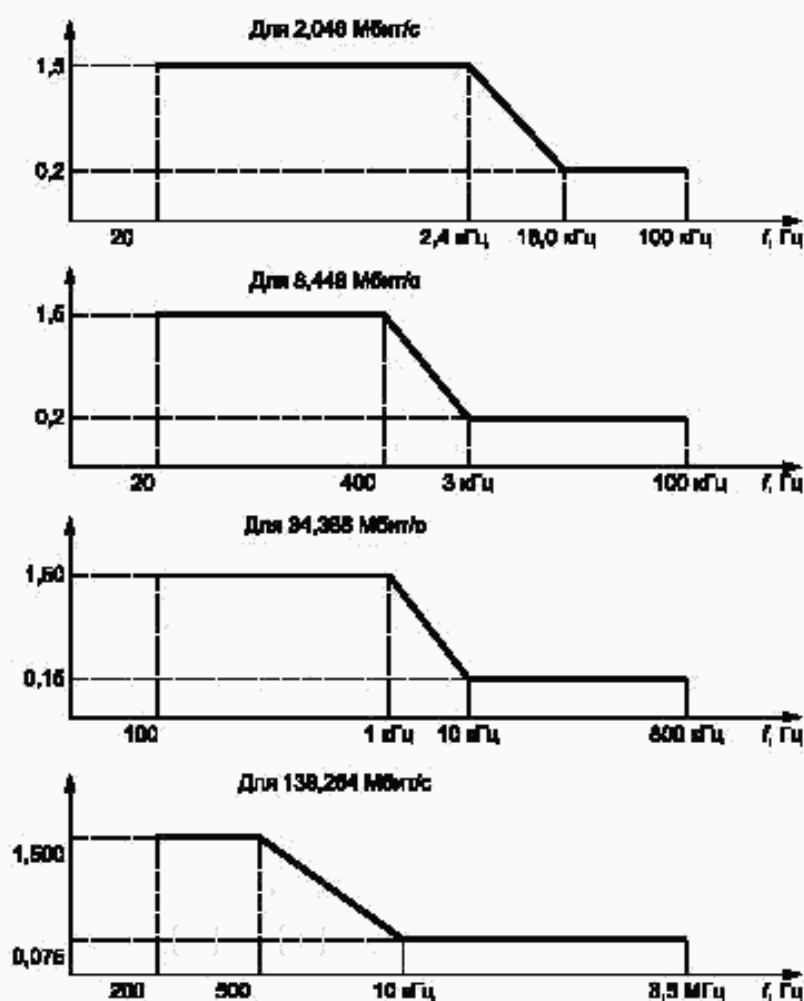
Рисунок 4.16 — Маски сигналов с предельным фазовым дрожанием
