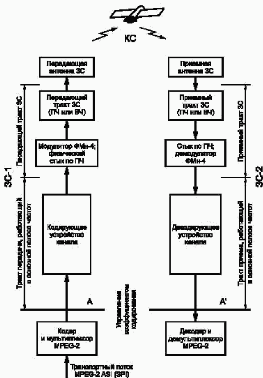
Рисунок 4.10 — Структурная схема СПТ передачи сигналов ЦТВ
