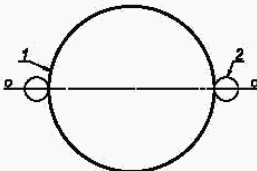
1 — труба; 2 — замок; O — O — ось шпунтовой стены
