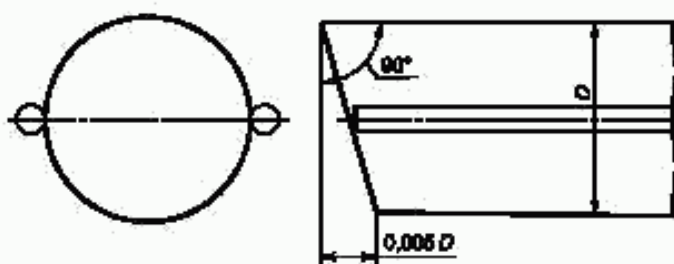
Рисунок 6 — Предельный перекосяк плоскости торца шпунтового профиля
