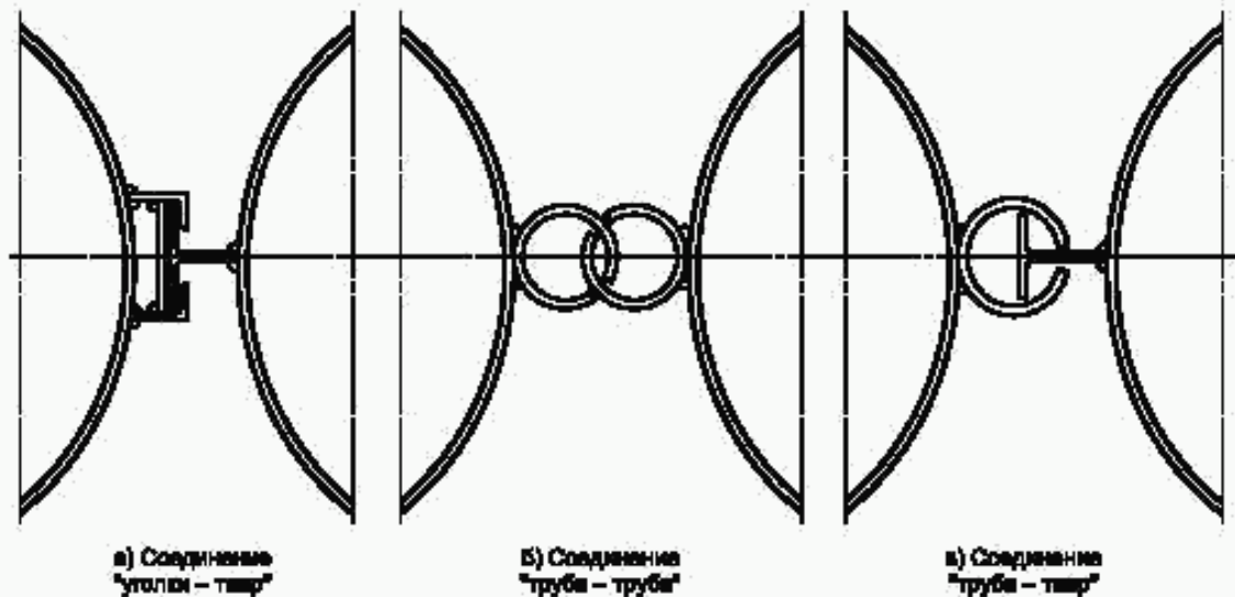
Рисунок 3 — Предпочтительные типы замковых соединений шпунтовых профилей
