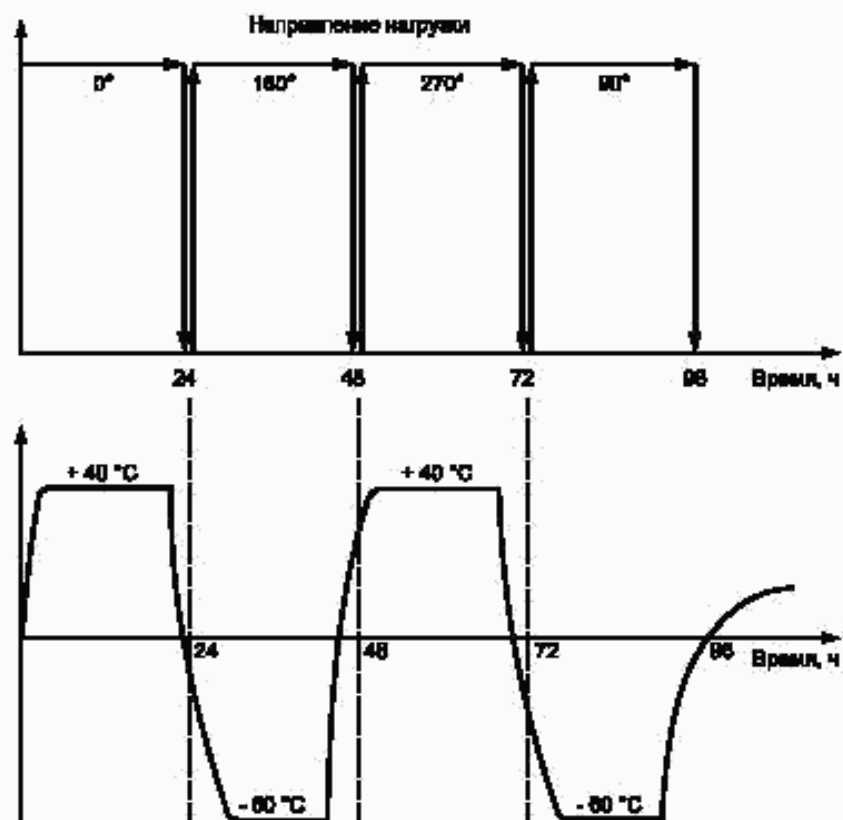
Рисунок 4 — Термомеханические испытания
