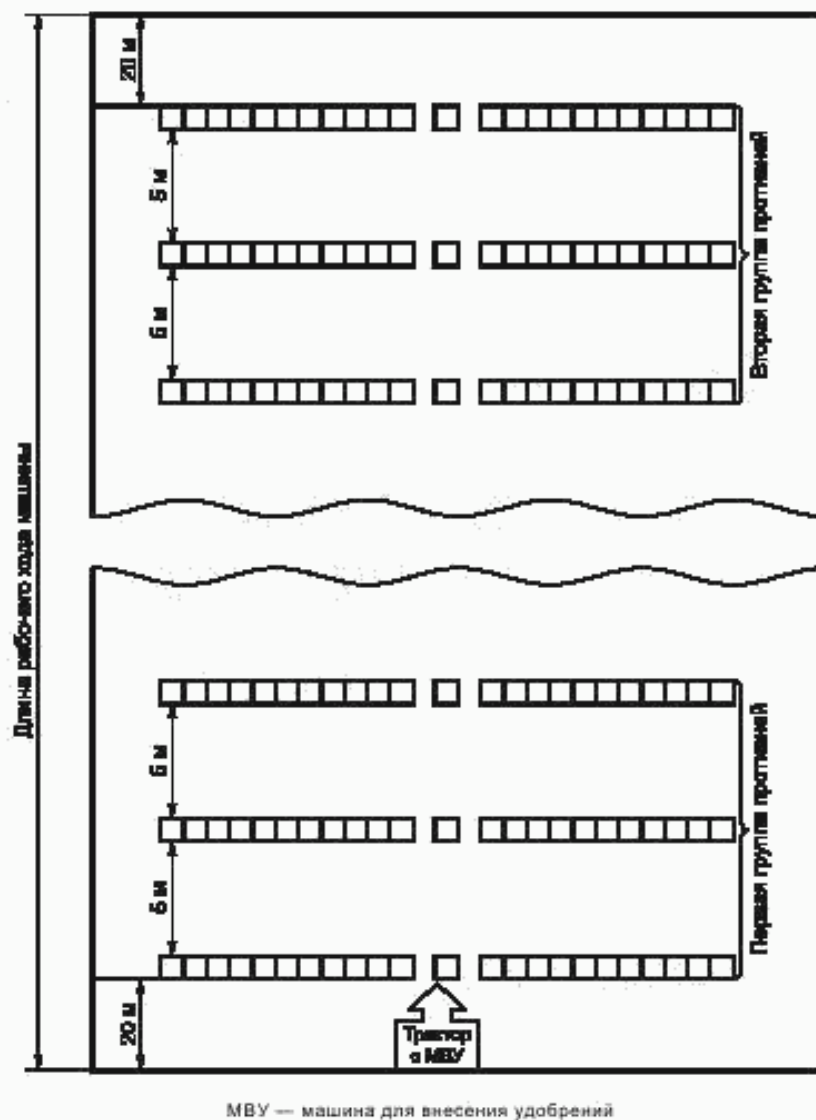
Рисунок 3 — Схема размещения контейнеров одной повторности при определении нестабильности дозы внесения удобрений
