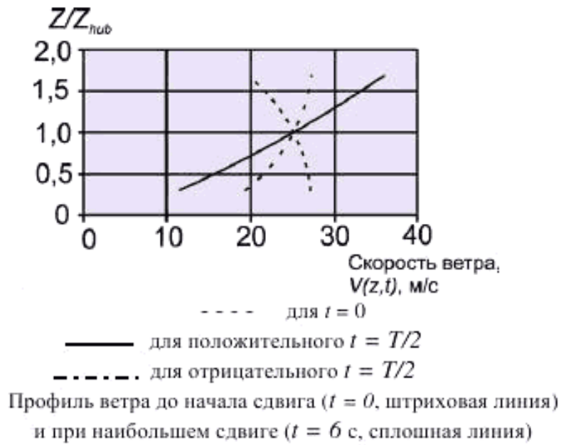
Рисунок 8 – Пример экстремального положительного и отрицательного вертикального сдвига ветра
