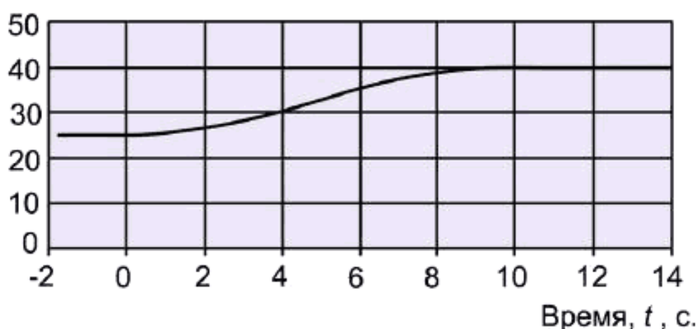
Рисунок 5 – Пример экстремального когерентного порыва с изменением амплитуды порыва для ЭЖН
