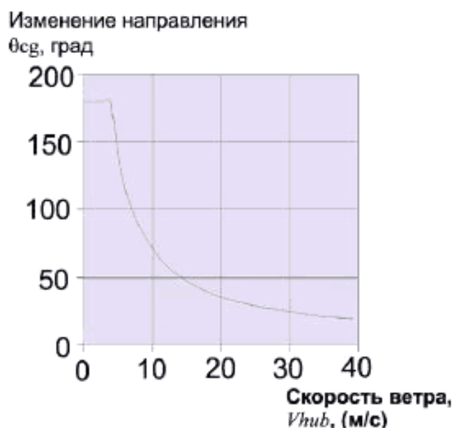
Рисунок 6 – Изменение направления для ЭКН
