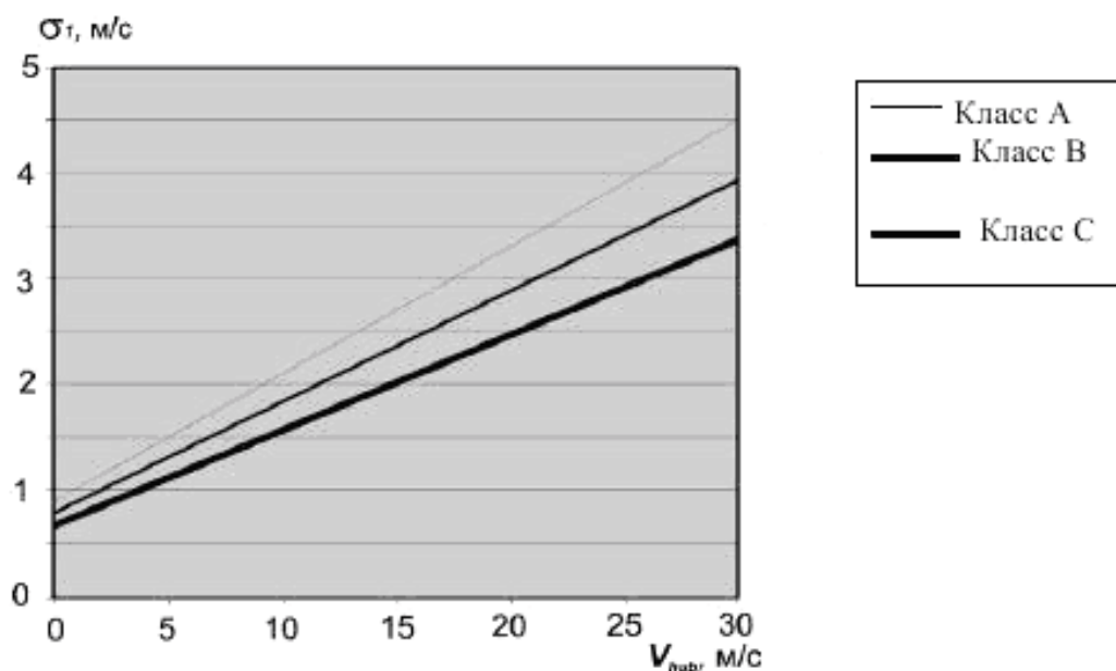
1а) – Среднее квадратическое отклонение продольной составляющей скорости ветра для модели НМТ
