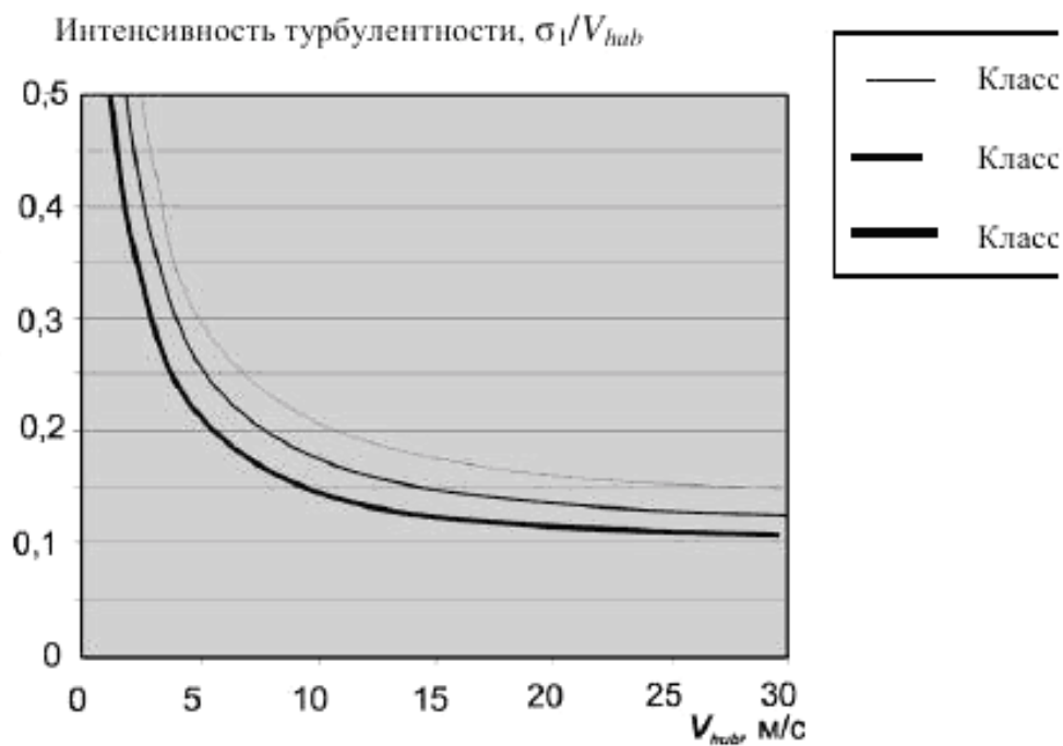
1б) – Интенсивность турбулентности для модели НМТ
