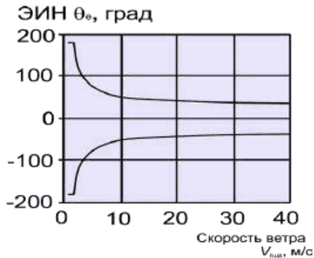
Рисунок 3 – Пример экстремальной величины изменения направления
