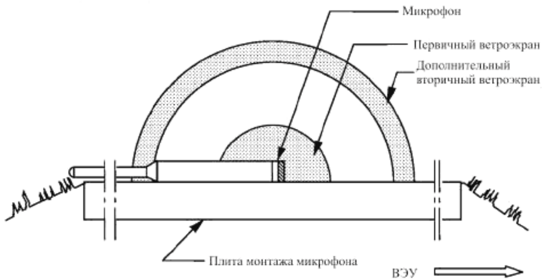
Рисунок 1б – Монтаж микрофона (вид сбоку)
