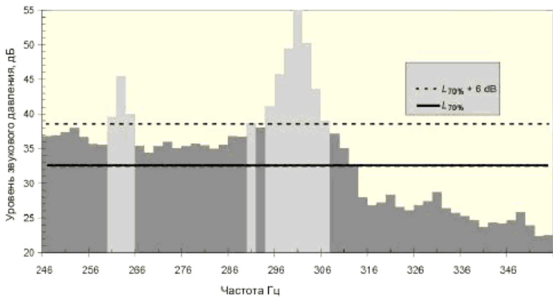
Рисунок 9 – Иллюстрация линий ниже критерия L_{70\%} + 6 дБ
