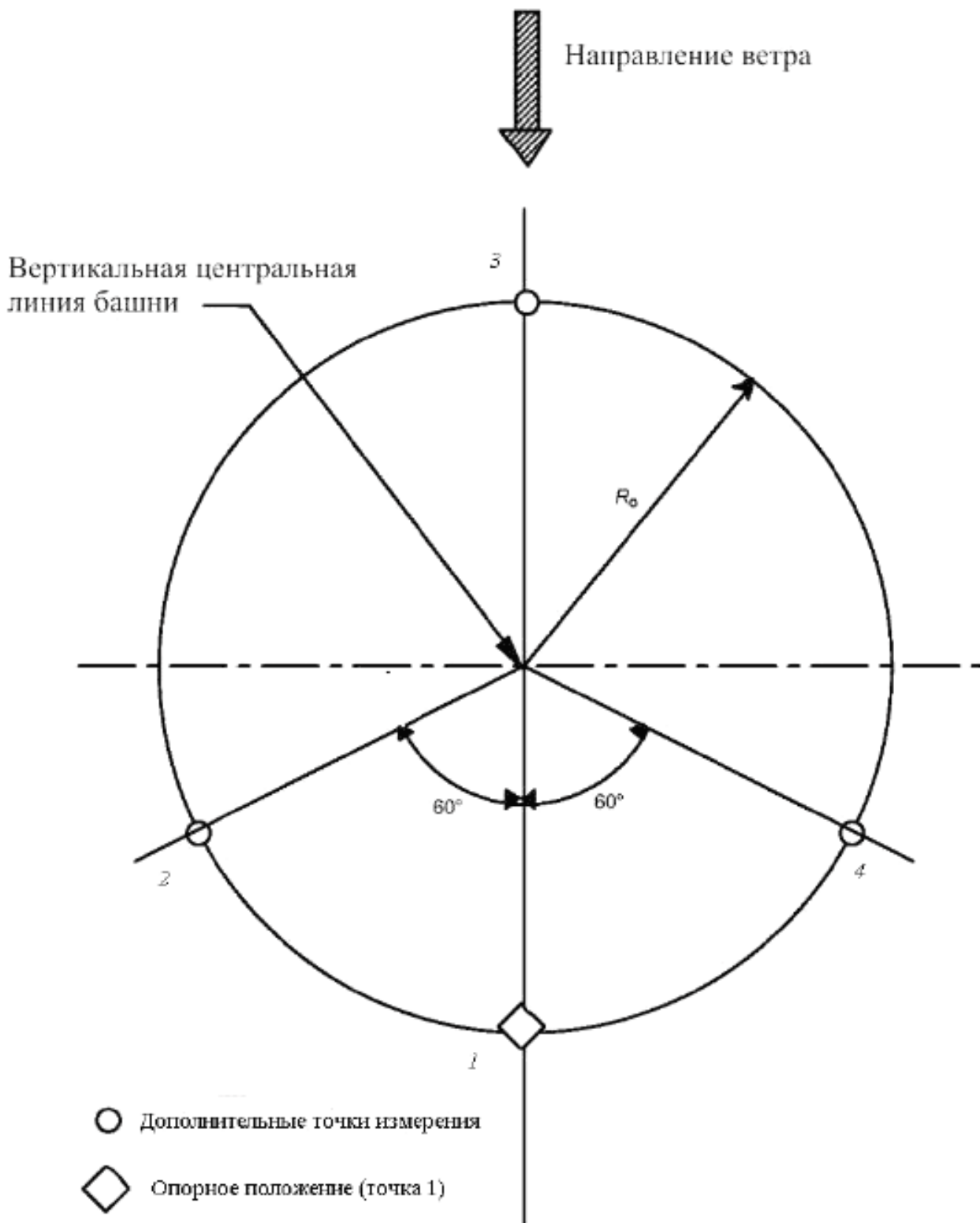
Рисунок 3 – Стандартная схема мест расположения микрофонов (вид сверху)
