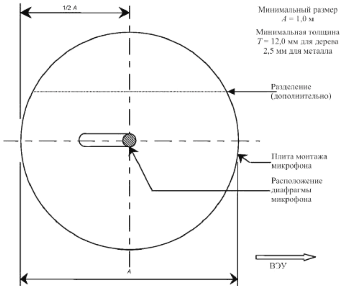
Рисунок 1а – Монтаж микрофона (вид сверху)
