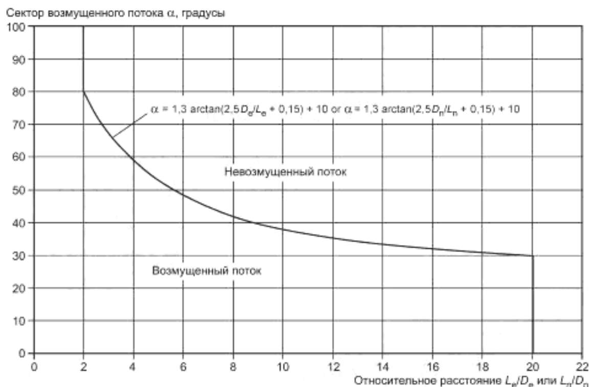
Рисунок А.1 — Секторы, которые необходимо исключить из-за возмущенного воздушного потока, вызванного соседней работающей ВЭУ и значительными аэродинамическими препятствиями
