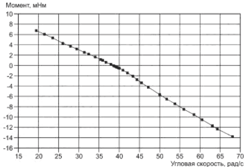
Рисунок J.2 — Измерения крутящего момента на чашечном анемометре в аэродинамической трубе при 8 м/с
