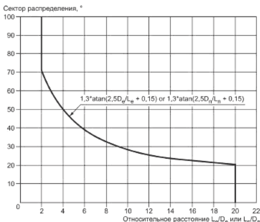
Рисунок Б.1 — Сектора, которые необходимо исключить из-за слутного следа соседних и работающих ВЭУ и значительных препятствий
