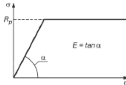
Рисунок 8 — Идеализированная зависимость упругой/пластичной деформации от напряжения
