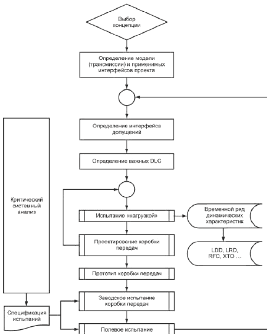
Рисунок 4 — Схема производственного процесса
