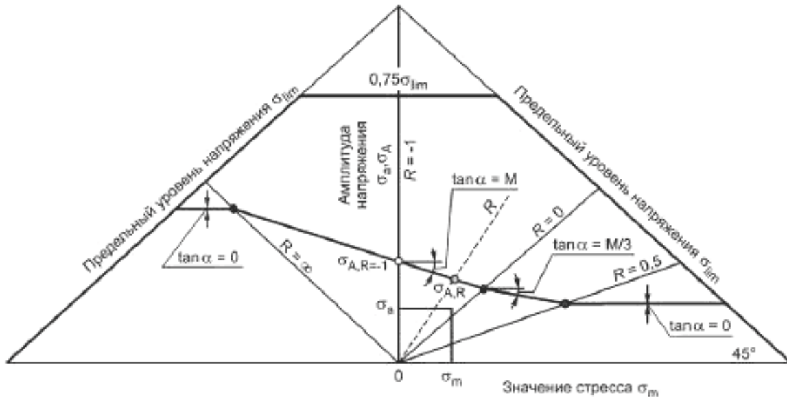
Рисунок 32 — Найг-диаграмма (цикла нагружения) для оценки влияния среднего напряжения
