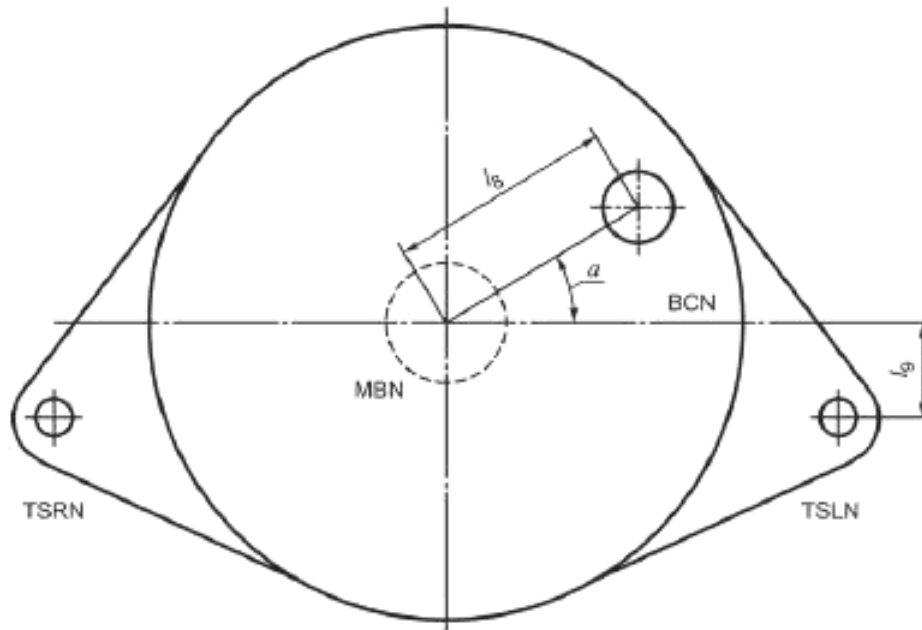
Рисунок 14 — Вид трансмиссии сзади
