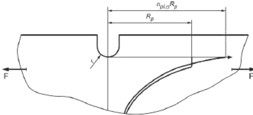
Рисунок 7 — Определение параметра секции n_{pl,\sigma} компонента с пазом
