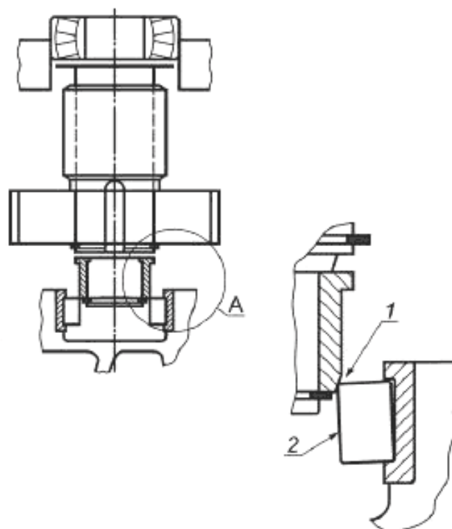
Вид А
