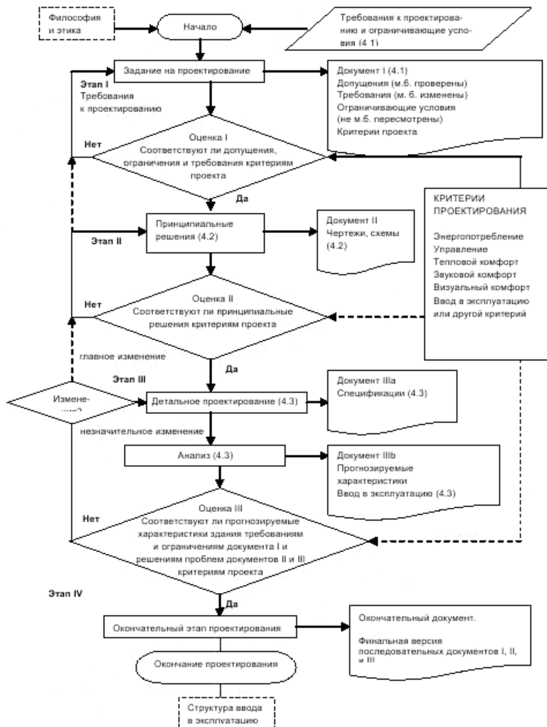
Рисунок А.1 — Диаграмма процесса проектирования
