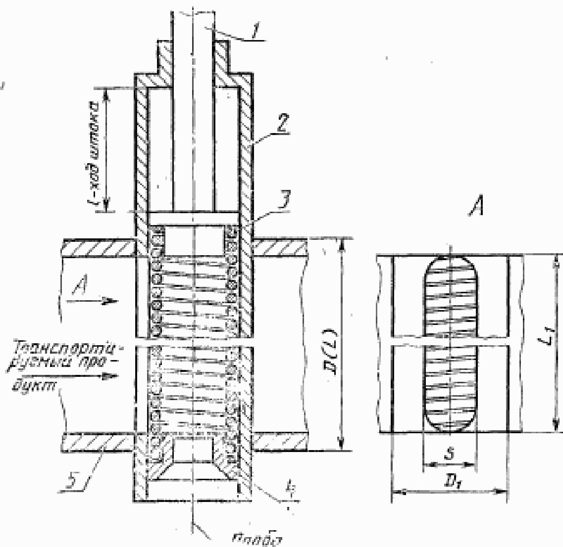
1 — шток; 2 — труба; 3 — пробоотбирающий элемент; 4 — воронка; 5 — трубопровод
