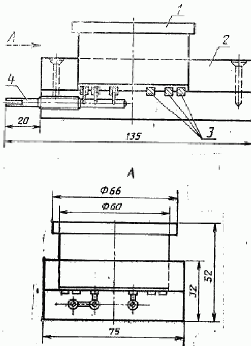
1 — крышка; 2 — корпус; 3 — кольца-конденсаторы; 4 — датчики
