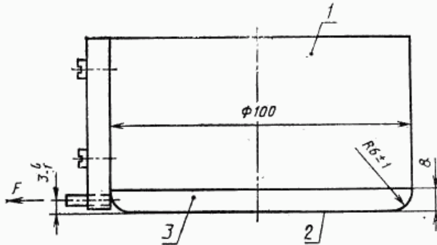
Рисунок 2 — Фрикционный цилиндр
