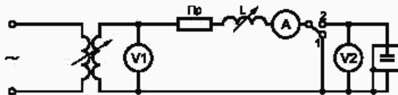
Pr — тугоплавкий предохранитель; L — регулируемая катушка индуктивности; V1 и V2 — вольтметры; A — амперметр
