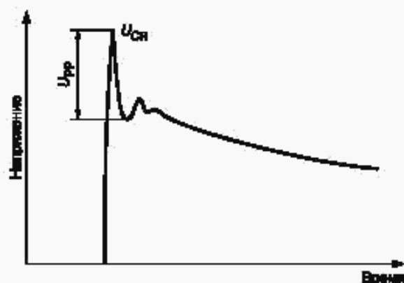
Рисунок 6 — Форма импульса
