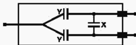
Рисунок 5b — Шунтирующий конденсатор, соединенный по схеме треугольника
