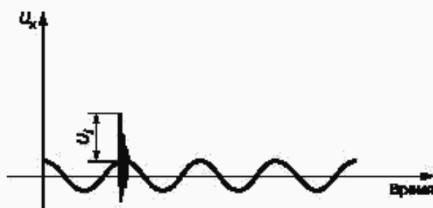
U_x — напряжение, прикладываемое к конденсатору C_x ; U_p — пиковое напряжение
