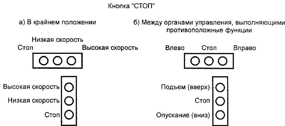
Рисунок 4 — Кнопка «СТОП» в наборе органов управления
