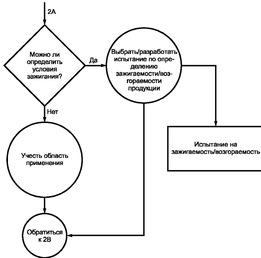
Рисунок А.3 — Блок-схема 2А. Зажигаемость/возгораемость
