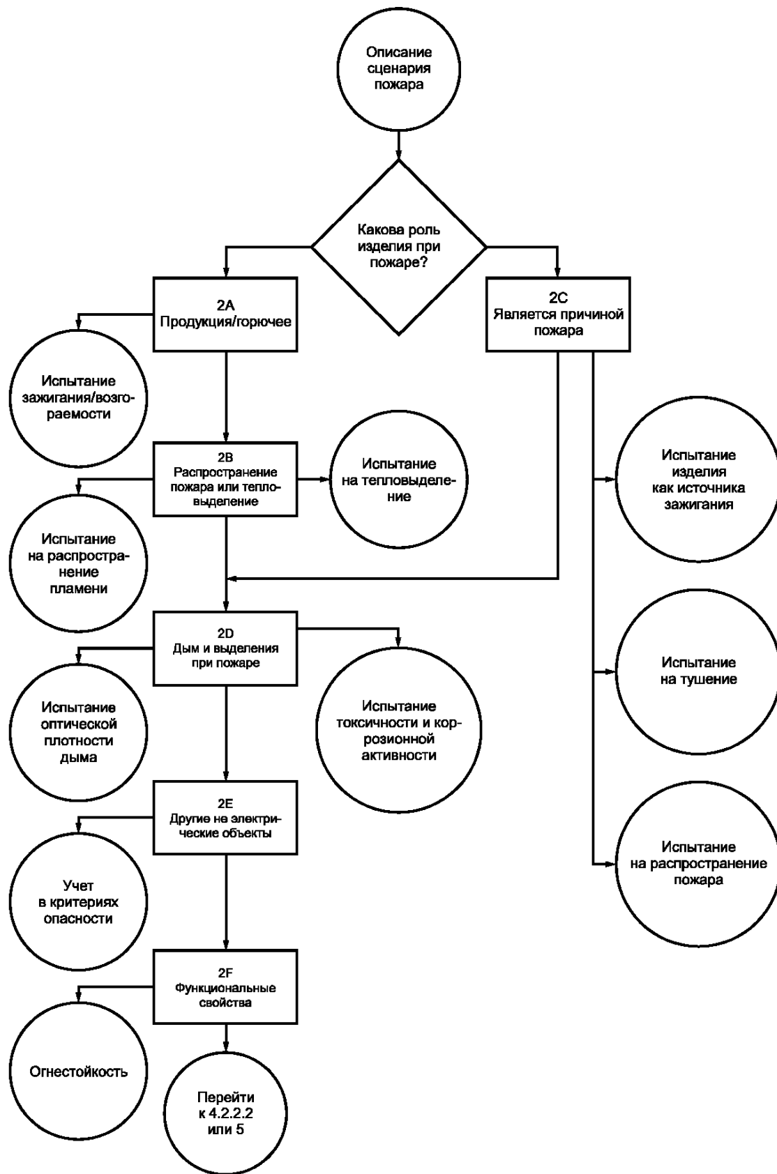
Рисунок А.2 — Блок-схема 2. Описание сценария пожара
