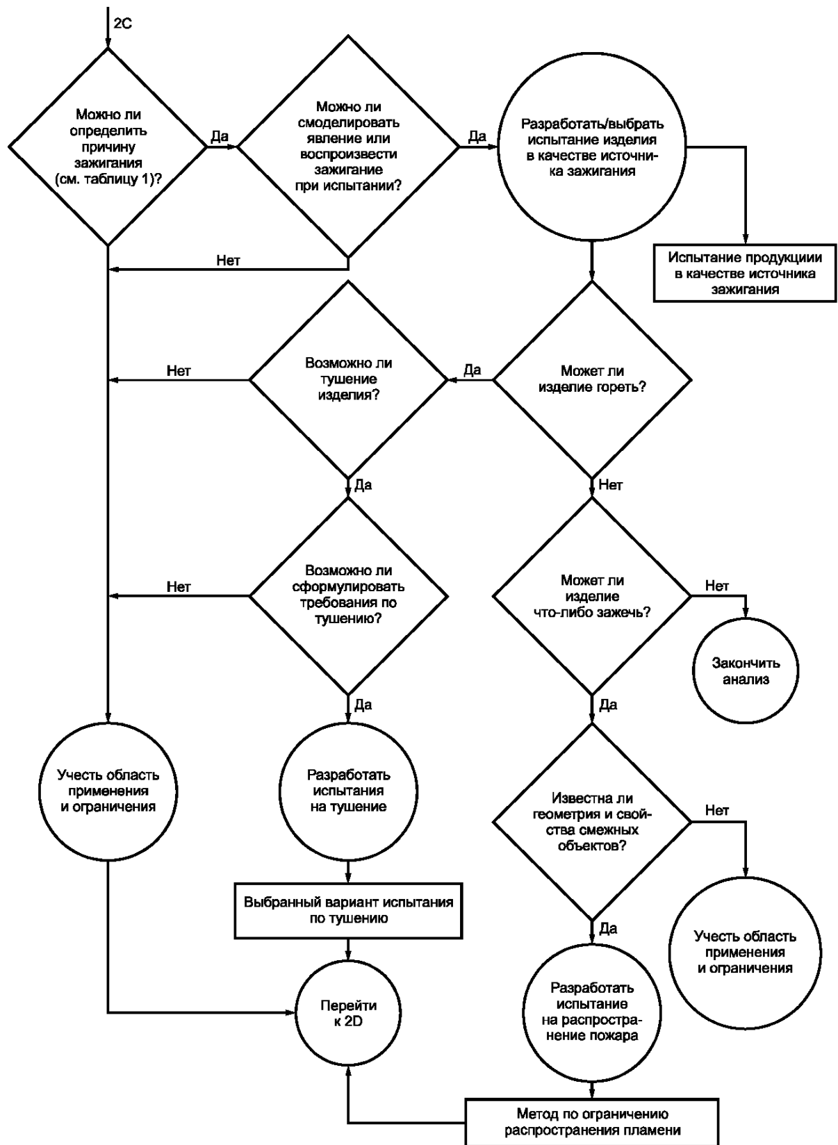
Рисунок А.5 — Блок-схема 2С. Причина пожара
