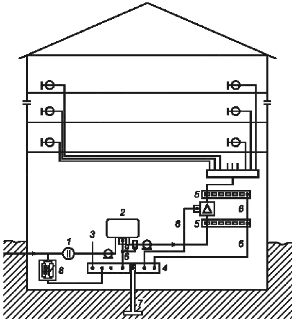
1 — гальванический изолятор; 2 — узел сопряжения, 3 — защитный проводник (РЕ), если необходим; 4 — заземляющий электрод; 5 — шина уравнивания потенциалов а ; 6 — защитный уравнивающий проводник (минимальное сечение согласно перечислению с) 6.2); 7 — заземляющий электрод; 8 — устройство защиты от перенапряжения (минимальное сечение уравнивающего проводника, идущего к главной шине заземления 4, должно быть 16 мм 2 ; 9 — зажим заземления (см. перечисления), к) 6.2)
