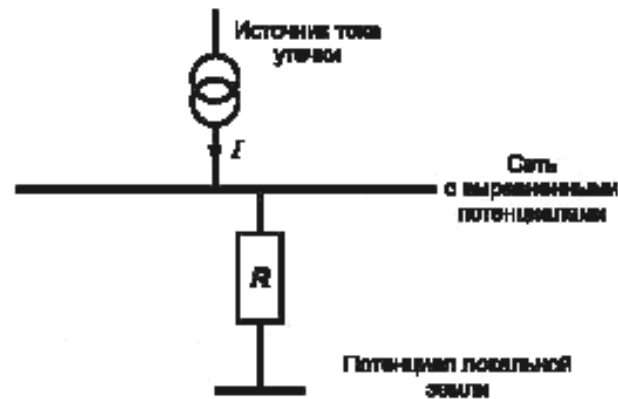
Рисунок А.1 — Сопротивление цепи заземления
