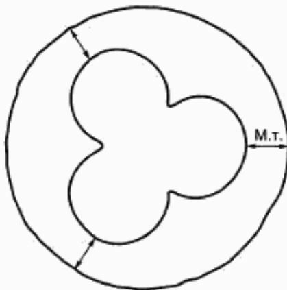
Рисунок 8 — Измерение оболочки (внутренний профиль некруглой формы)
