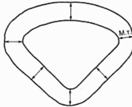
Рисунок 2 — Измерение толщины изоляции (секторная жила)
