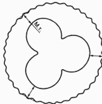
Рисунок 9 — Измерение толщины оболочки (наружная поверхность неправильной формы)
