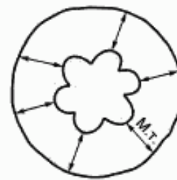
Рисунок 4 — Измерение толщины изоляции (многопроволочная жила)
