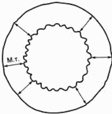
Рисунок 3 — Измерение толщины изоляции (многопроволочная жила)
