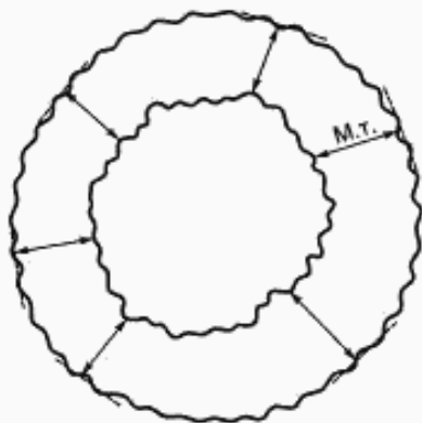
Рисунок 5 — Измерение толщины изоляции (неровный наружный профиль)
