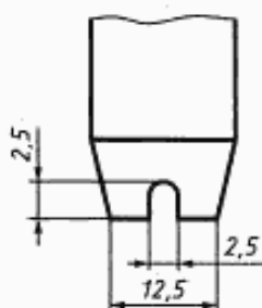
Рисунок 14 — Конеч вырубного ножа с выемкой
