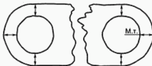
Рисунок 11 — Измерение толщины оболочки (плоский кабель с разделенными жилами)
