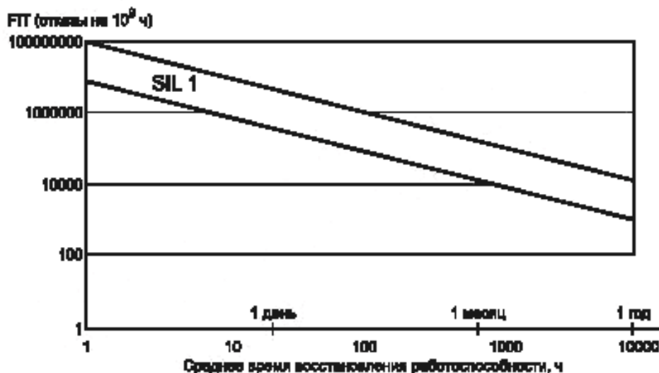
Рисунок D.4 — Диаграмма FIT и среднего времени восстановления работоспособности
