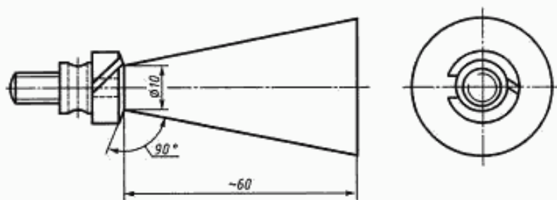
Рисунок 1 — Коническая оправка
