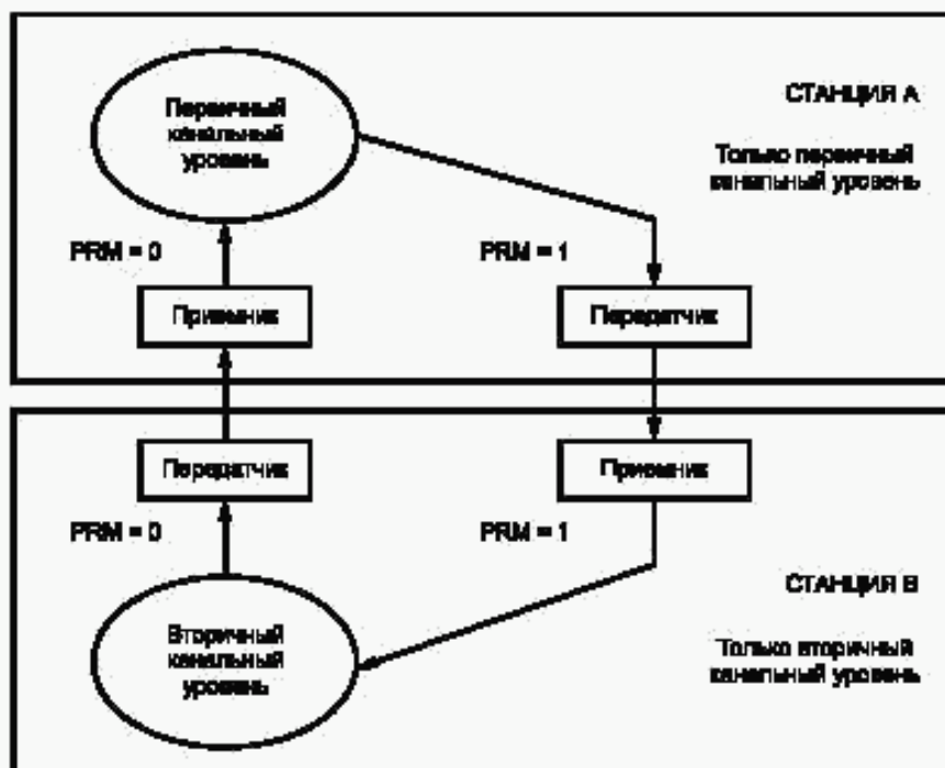
Рисунок 4 — Небалансные процедуры передачи, первичный и вторичный канальные уровни
