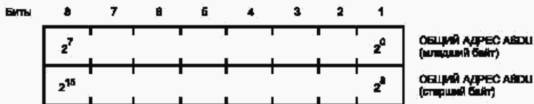
Рисунок 18 — ОБЩИЙ АДРЕС ASDU (два байта)
