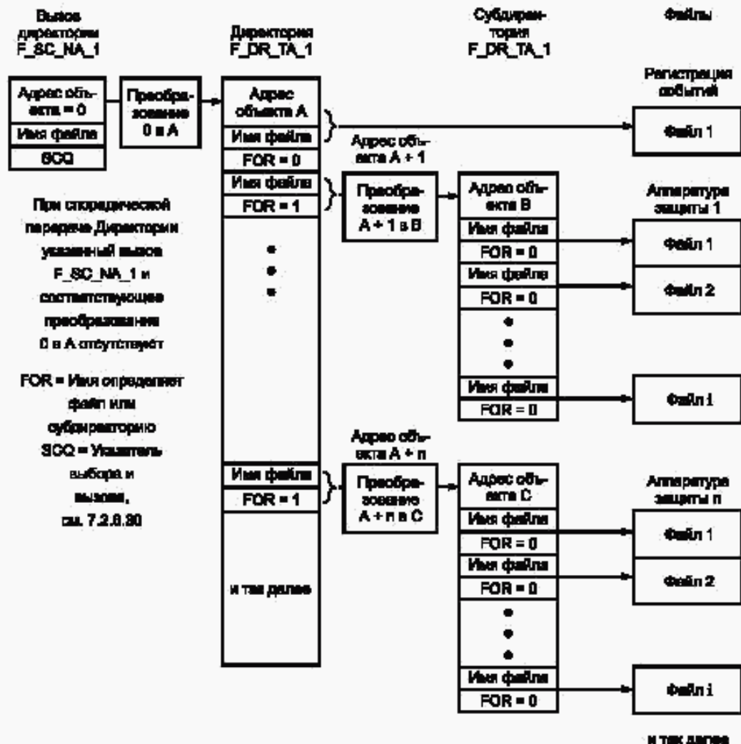
Рисунок 97 — Адресация файлов (пример)
