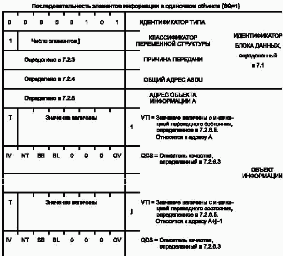
Рисунок 29 — ASDU: M_ST_NA_1 Последовательность информации о положении отпаяк
