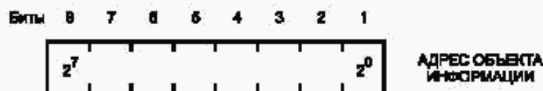
Рисунок 19 — АДРЕС ОБЪЕКТА ИНФОРМАЦИИ (один байт)
