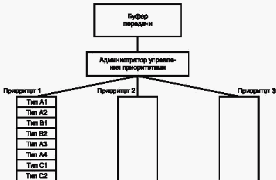
Рисунок 13 — Представление типов объектов информации в приоритетных буферах
