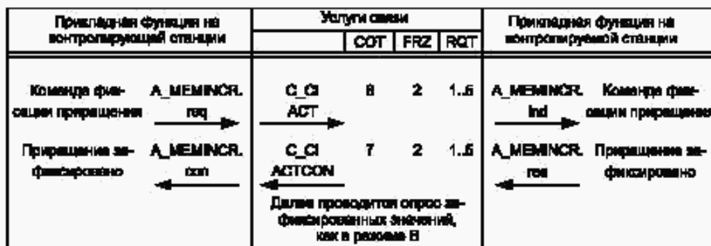
Рисунок 96 — Последовательная процедура запоминания интегральных сумм со сбросом (Режим С)
