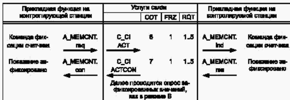
Рисунок 95 — Последовательная процедура запоминания интегральных сумм без сброса (Режим С)
