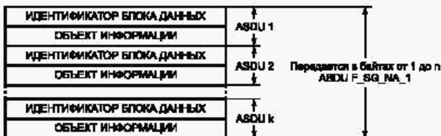
Рисунок 105 — Запись последовательности событий в секции файла данных
