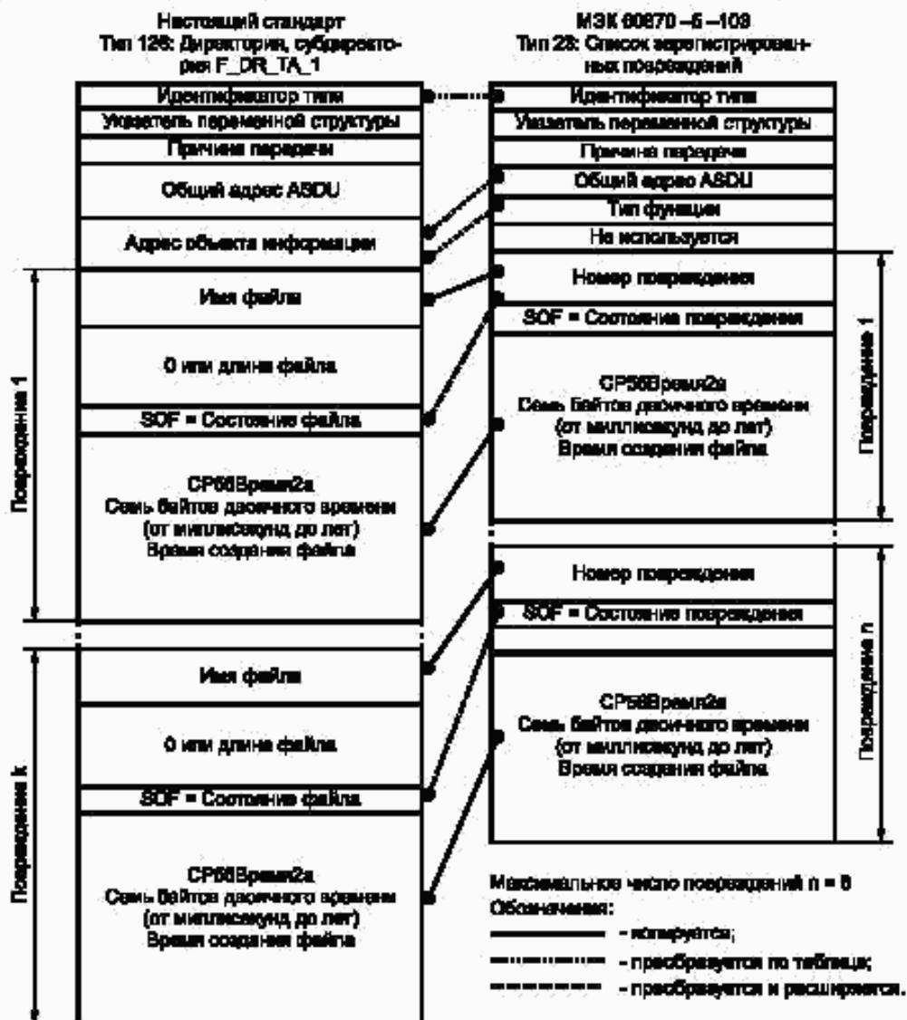
Рисунок 102 — Преобразование блока данных типа 23 в директорию F_DR_TA_1
