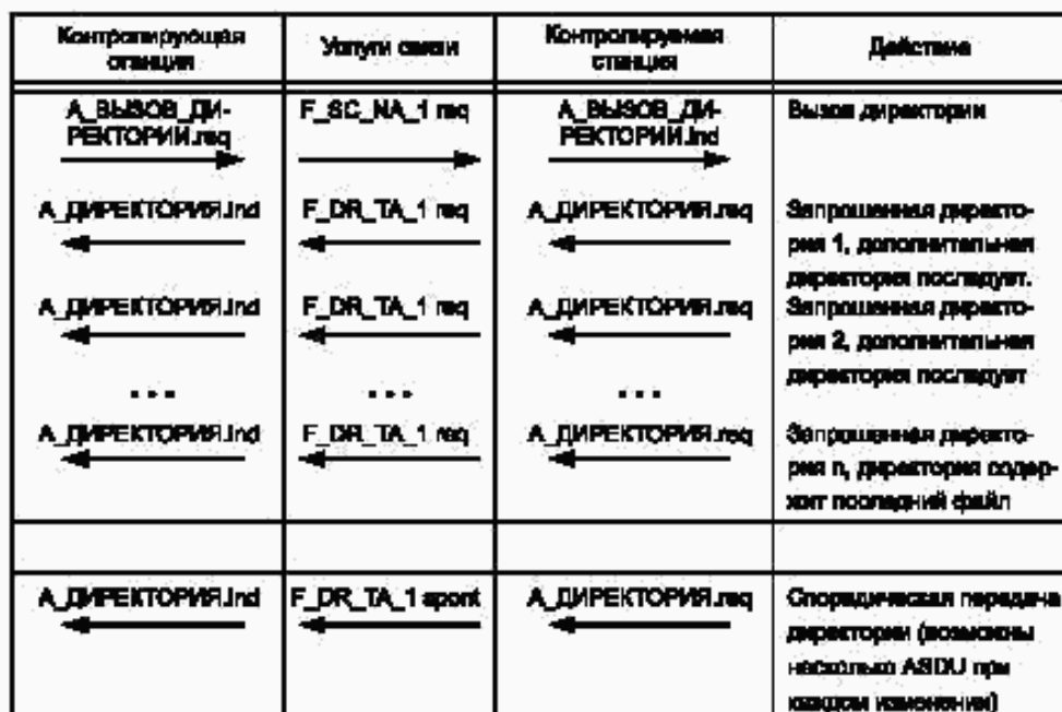
Рисунок 103 — Последовательная процедура передачи директории
