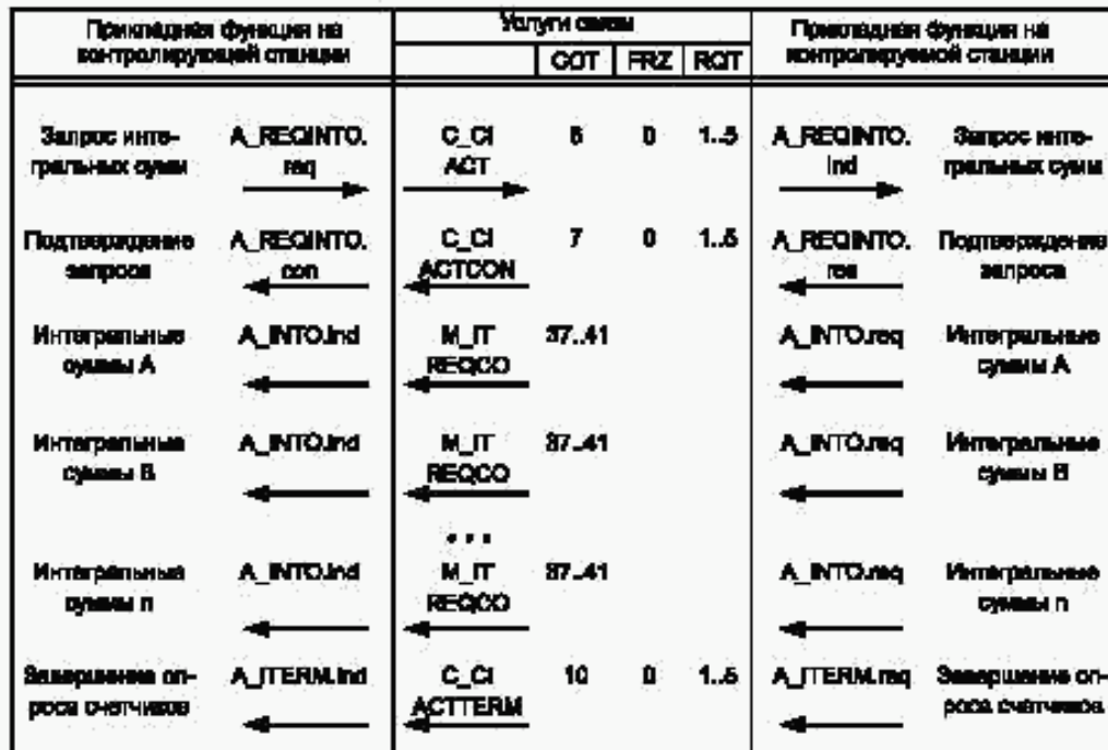
Рисунок 94 — Последовательная процедура опроса интегральных сумм (Режим В)
