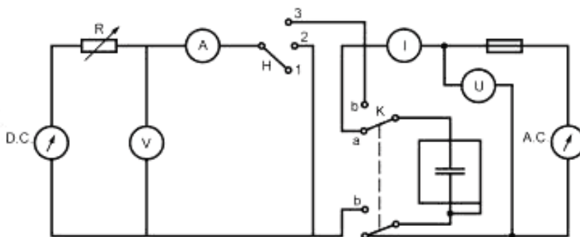
Рисунок 1 — Электрическая схема для выполнения испытания на разрушение
