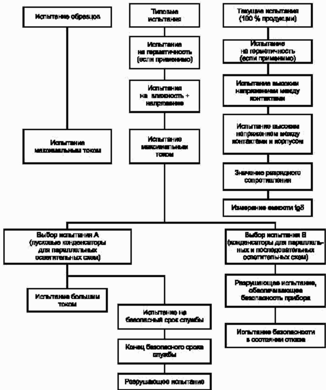
Рисунок 4— Схема процедуры испытаний
