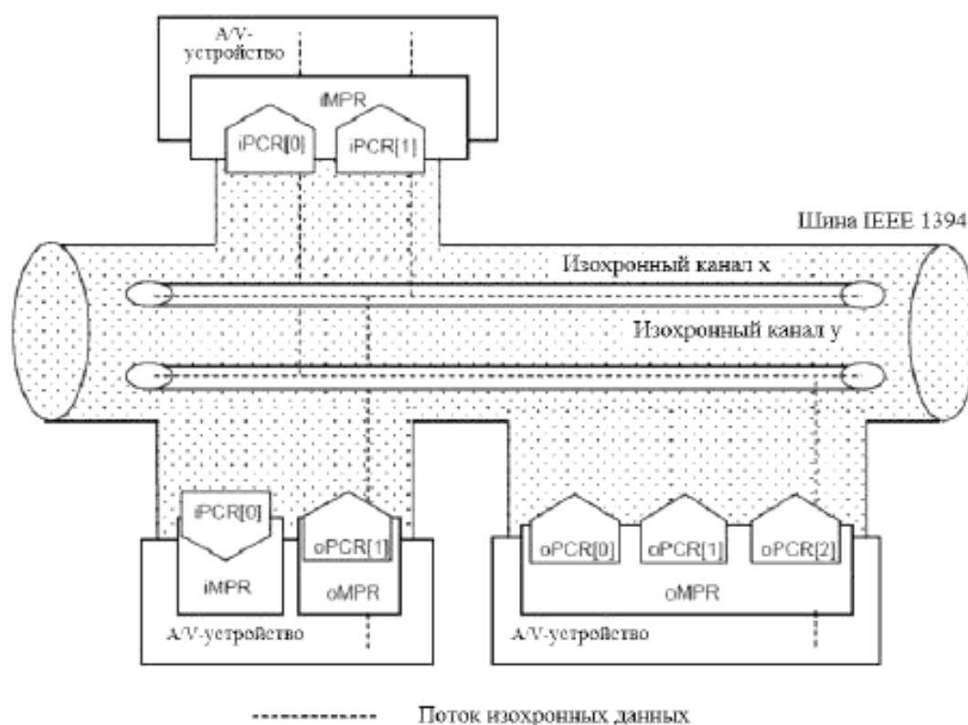
Рисунок 7 – Использование разъемов и регистров управления разъемами
