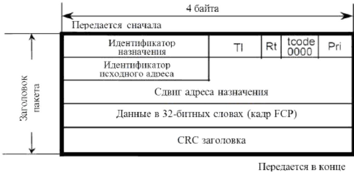
Рисунок 31 – Запрос записи для пакета квадлет данных IEEE 1394
