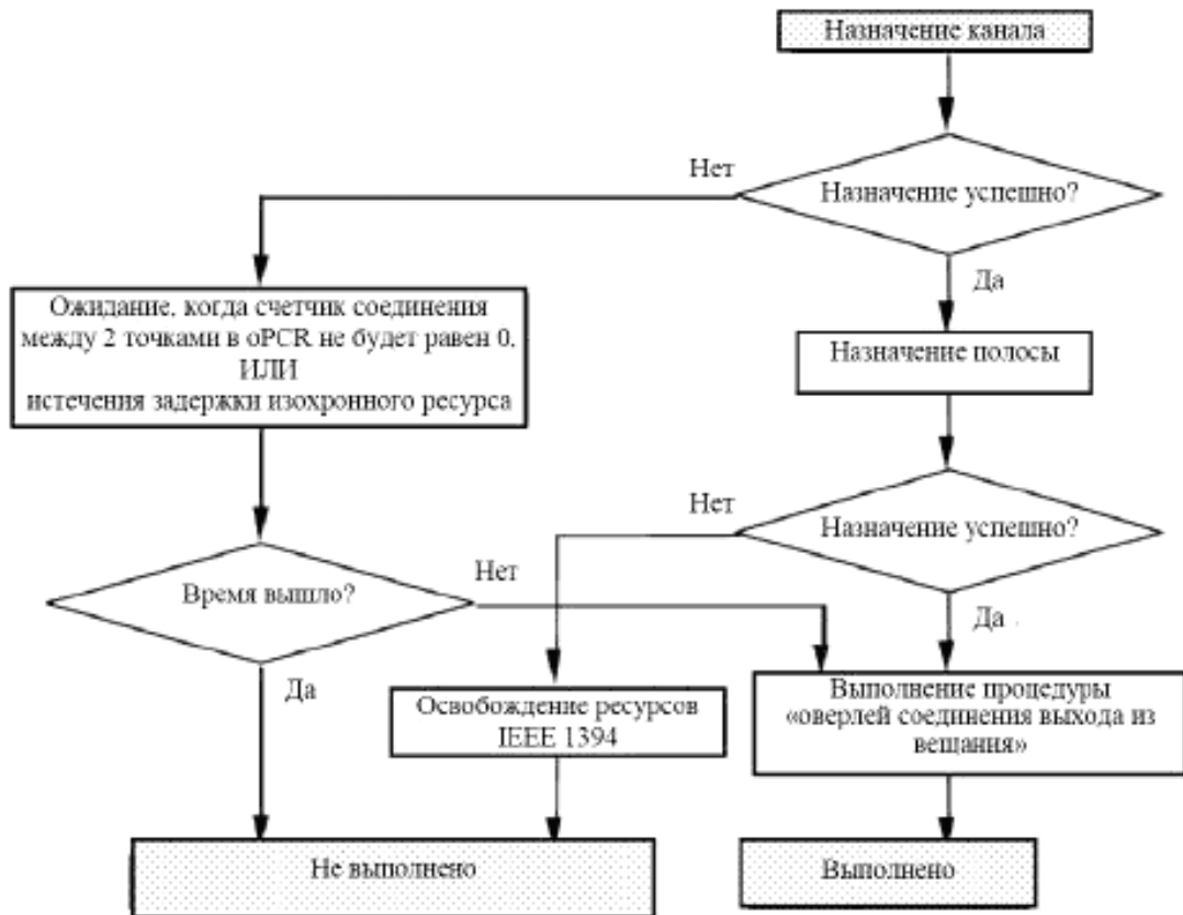
Рисунок 27 – Восстановление соединения выхода из вещания
