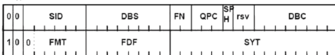
5а – Заголовок CIP с полем SYT
