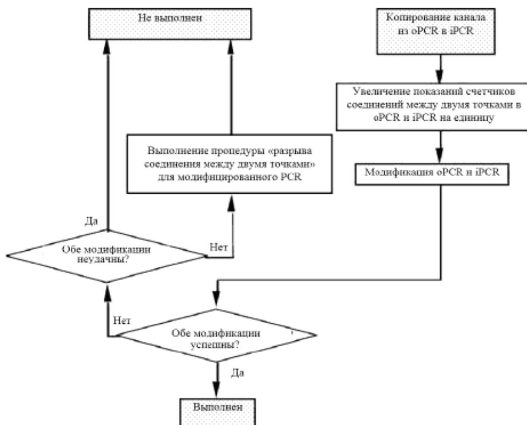
Рисунок 17 – Замена (наложение) соединения между двумя точками
