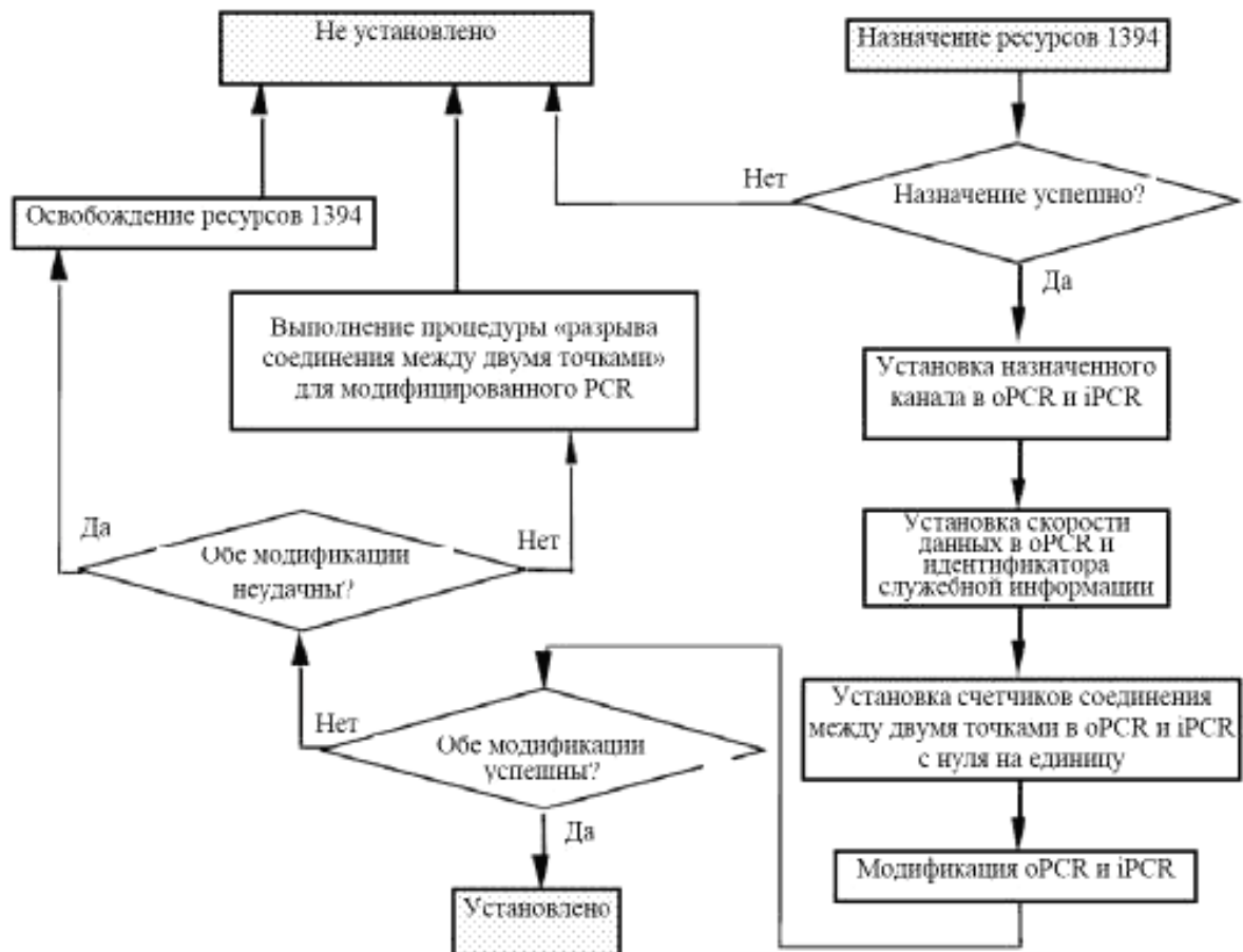
Рисунок 16 – Установка соединения между двумя точками
