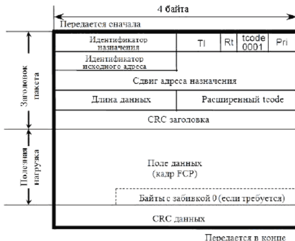
Рисунок 30 – Запрос записи для пакета блока данных IEEE 1394
