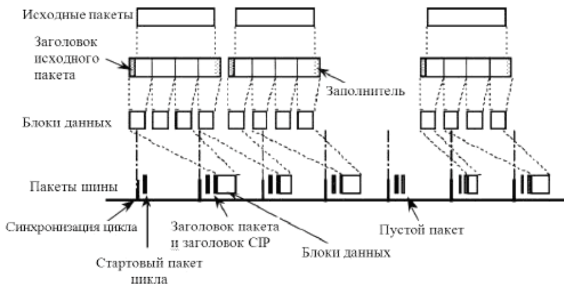
Рисунок 4 – Модель передачи исходных пакетов
