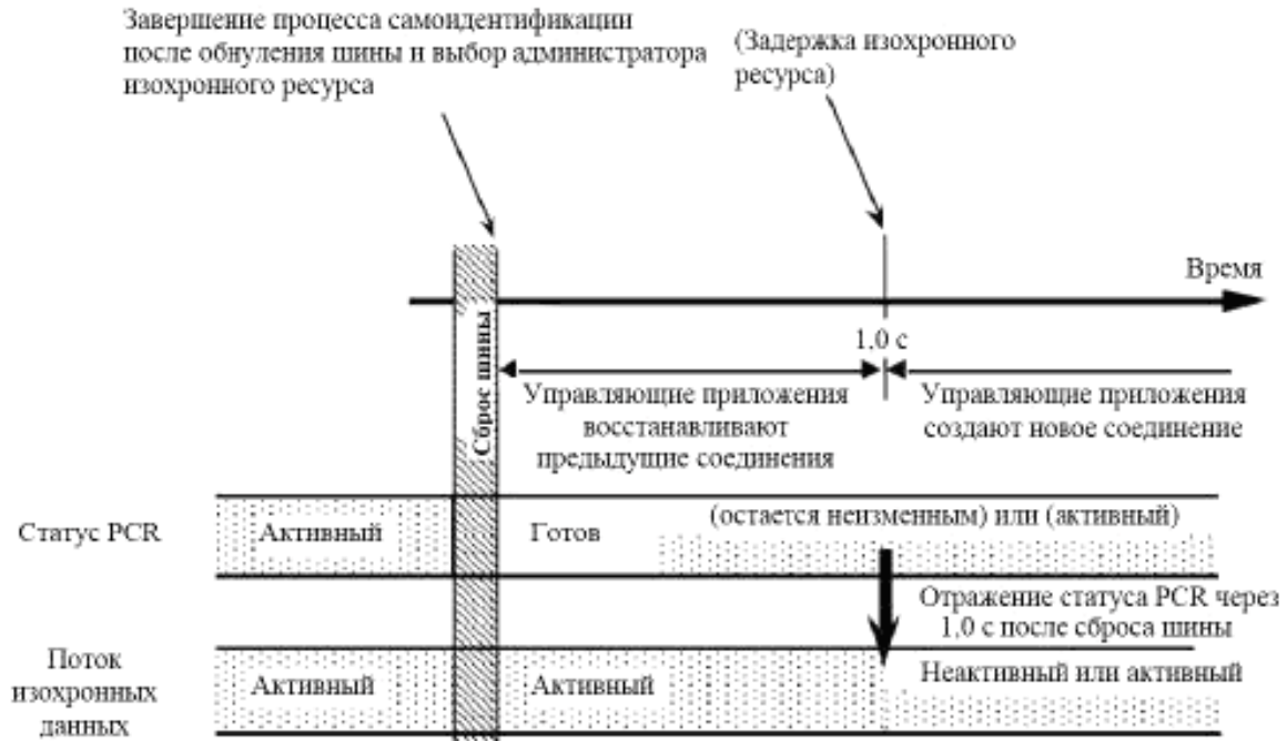
Рисунок 25 – Временная диаграмма управления соединениями и работа PCR
