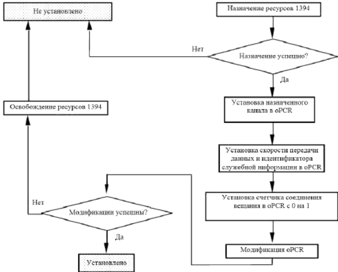
Рисунок 19 – Установка соединения выхода из вещания
