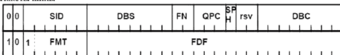
5б – Заголовок CIP без поля SYT
