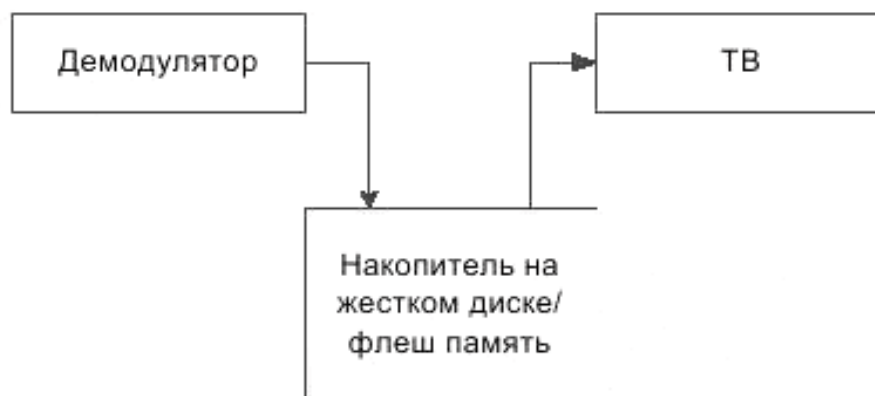
Рисунок D.2 – Регистрация временного сдвига с одним тюнером
