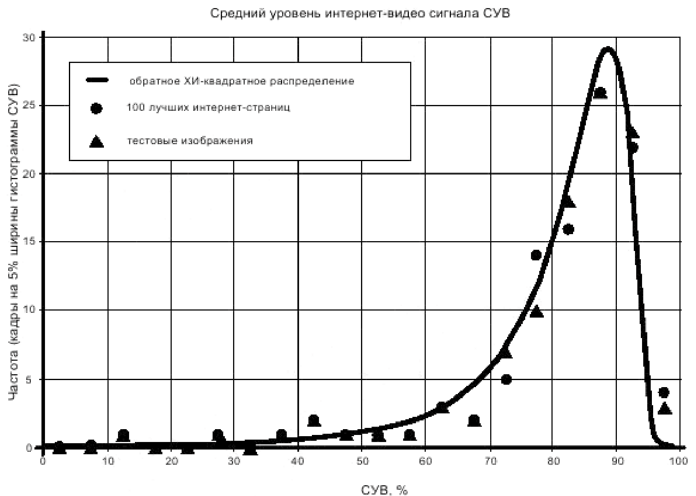
Рисунок С.2 – Средний уровень интернет-видеосигнала
