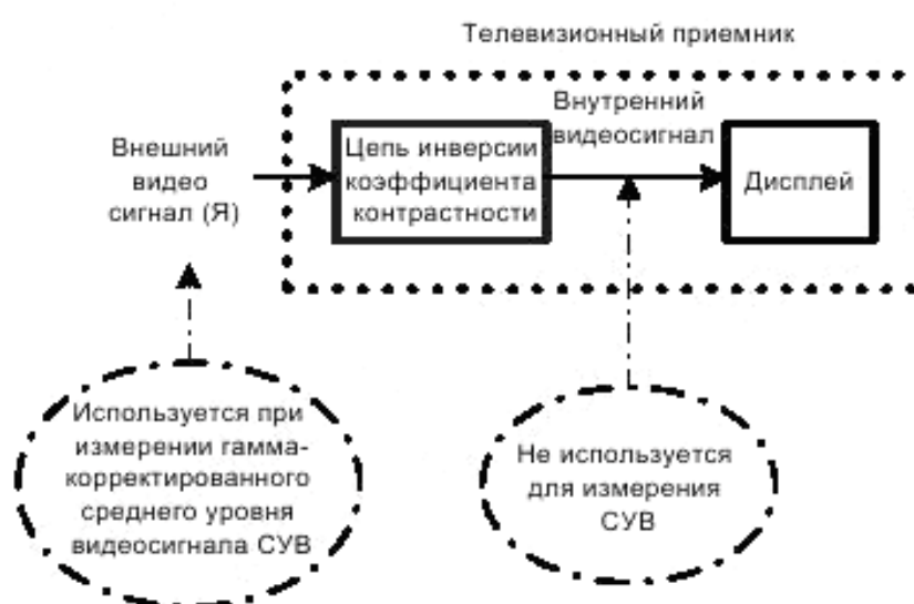
Рисунок 1 – Гамма-корректированный средний графический уровень
