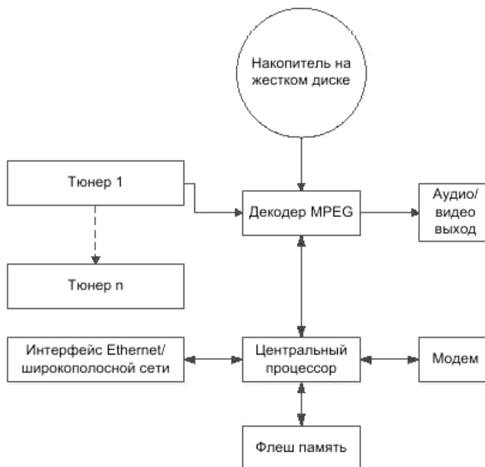
Рисунок D.1 Блок-схема основных функциональных частей РЦТ
