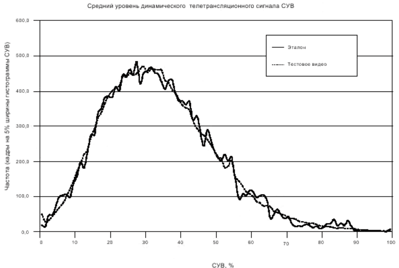
Рисунок С.1 – Средний уровень динамического телетрансляционного видеосигнала
