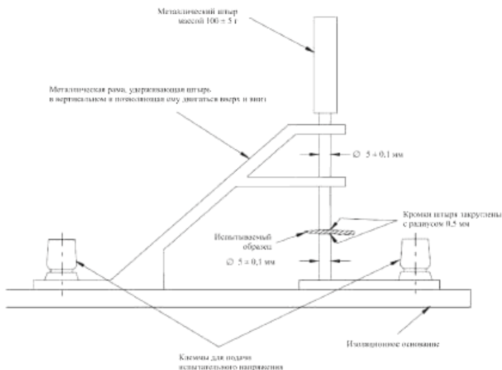
Р и с у н о к 36 – Пример установки для испытаний на электрическую прочность
