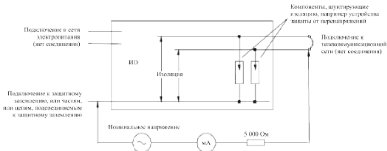
Р и с у н о к 37 – Испытание разделения между телекоммуникационной сетью и землей
