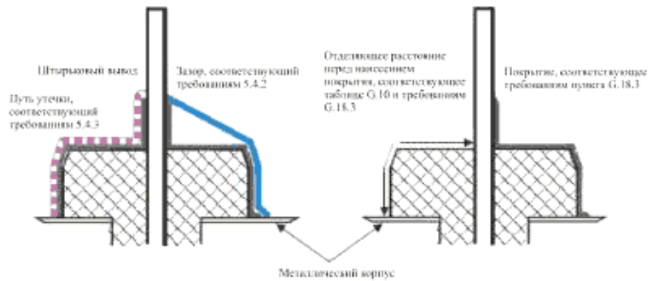
Р и с у н о к О.11 – Покрытие выводов
