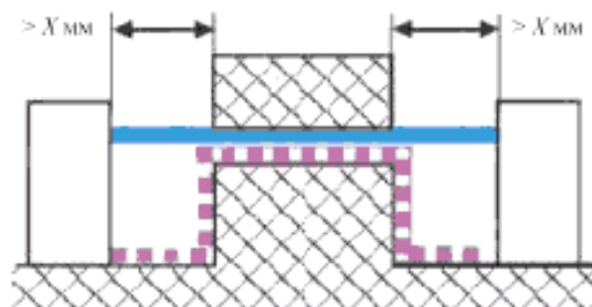
Р и с у н о к О.6 – Нескрепленный стык с узкой канавкой
