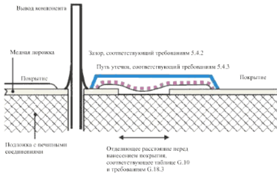
Р и с у н о к О.12 – Покрытие поверх печатного монтажа
