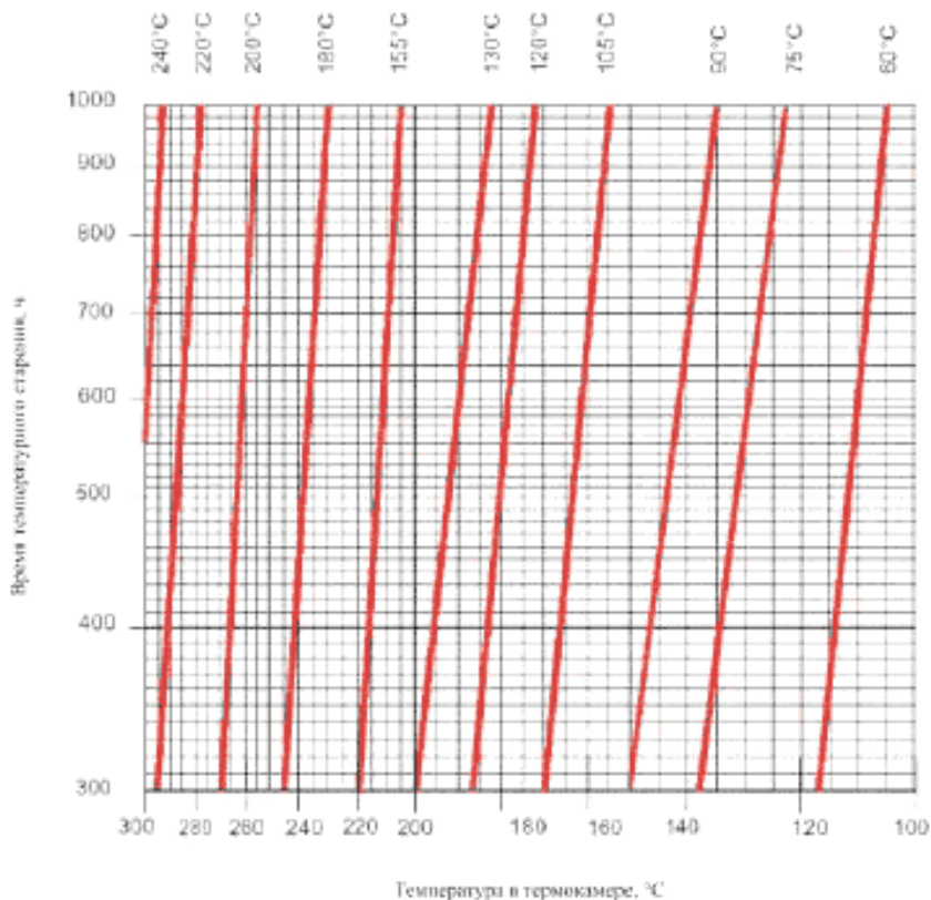
Р и с у н о к G.2 – Время теплового старения
