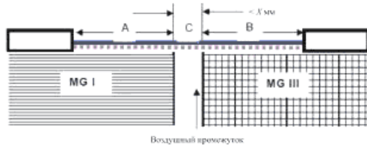
Р и с у н о к О.17 – Материалы с разными значениями СИТ
