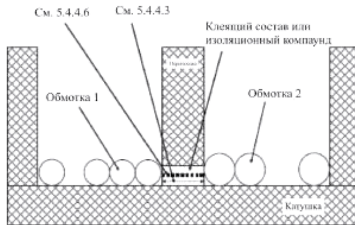
Р и с у н о к О.16 – Секционированная катушка
