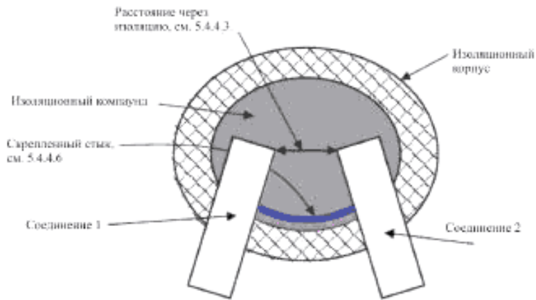
Р и с у н о к О.15 – Устройство, заполненное изоляционным компаундом
