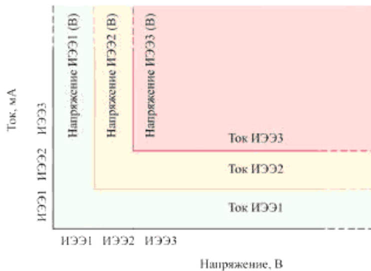
Р и с у н о к 23 – График, демонстрирующий, что предельные значения параметров ИЭЭ зависят и от тока, и от напряжения
