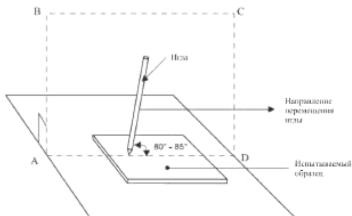
Р и с у н о к G.3 – Испытание слоев покрытия на абразивную изностоустойчивость
