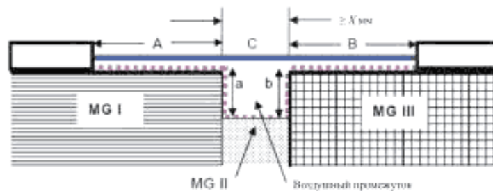
Р и с у н о к О.19 – Компоненты из материалов с разными значениями СИТ, воздушная канавка между которыми имеет ширину менее X мм
