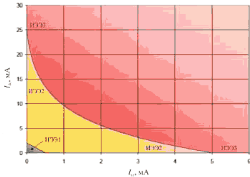
Р и с у н о к 24 – Максимальные значения переменного и постоянного тока для комбинированного источника
