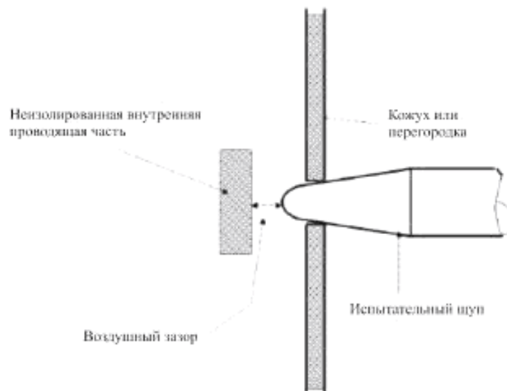
Р и с у н о к 31 – Требования по допустимости контакта с неизолированной внутренней проводящей частью
