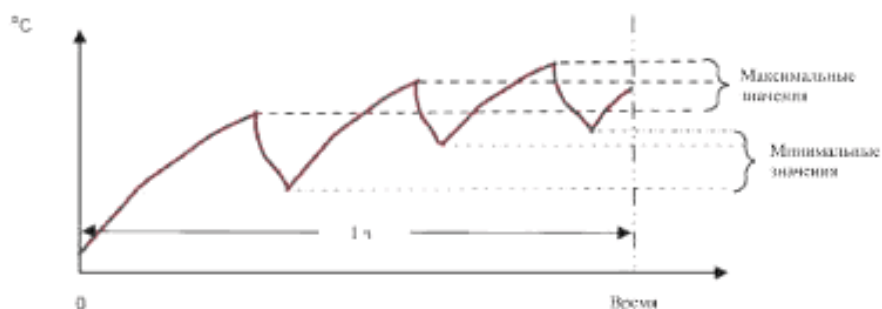
Р и с у н о к G.1 – Определение среднеарифметического значения температуры
