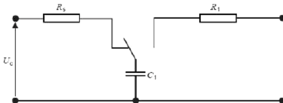
Р и с у н о к D.2 – Испытательный генератор для интерфейса антенны
