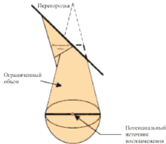
Р и с у н о к 44а – Наклонная перегородка
