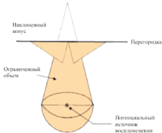
Р и с у н о к 44б – Горизонтальная перегородка
