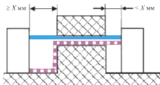
Р и с у н о к О.7 – Нескрепленный стык с широкой канавкой
