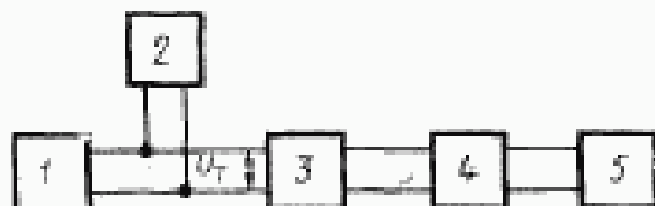
1 — звуковой генератор; 2 — вольтметр; 3 — телефон; 4 — прибор «искусственное ухо»; 5 — прибор для измерения коэффициента гармонических искажений телефона K_{г.и.т.} на высших гармониках.
