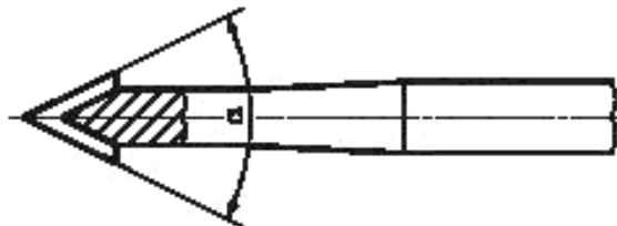
Рисунок 1 — Включенный (внутренний) угол для конусных алмазных инструментов
