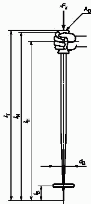
Рисунок 2 — Условное обозначение размеров горнолыжной палки
