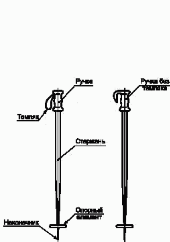
Рисунок 1 — Элементы горнолыжной палки и термины
