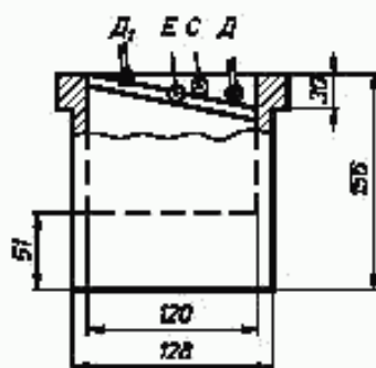
Рисунок 1 — Зональный пробоотборник
