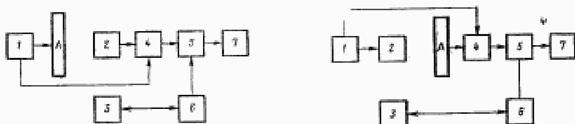
а. Испытуемая антенна в передающем режиме
