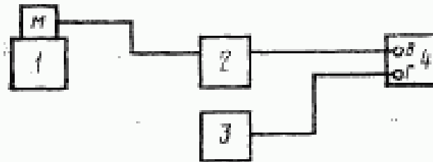
1—поверяемый хронометр; 2—преобразователь звуковых сигналов с микрофоном М; 3—кварцевый синхронизатор; 4—электронно-счетный частотомер
