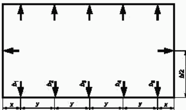
x = 200 мм; y \geq 1000 мм; b — среднее значение результатов измерений ширины
