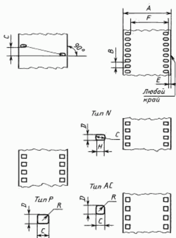
Типы перфораций
