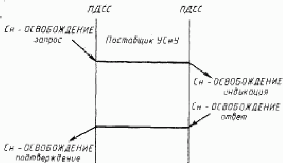
Рисунок 23 — Последовательность примитивов услуги Сн-ОСВОБОЖДЕНИЕ
