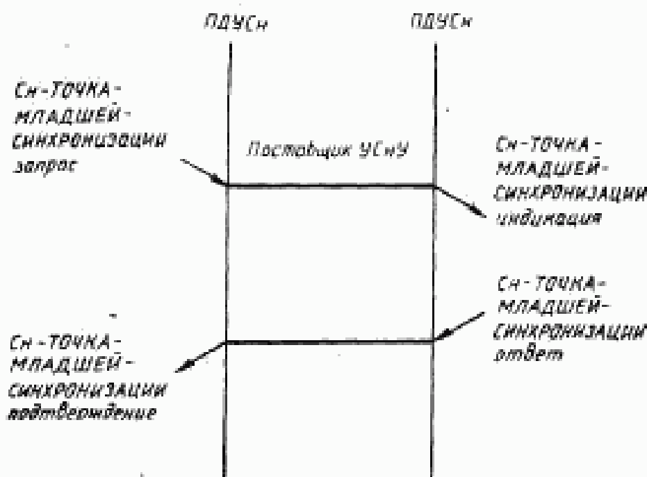
Рисунок 13 — Последовательность примитивов услуги Сн-ТОЧКА-МЛАДШЕЙ-СИНХРОНИЗАЦИИ
