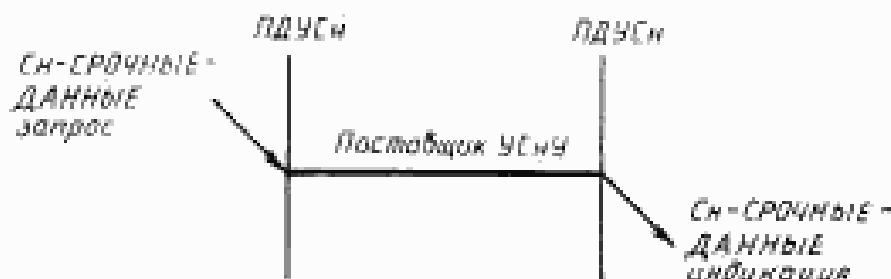
Рисунок 7 — Последовательность примитивов услуги Сн-СРОЧНЫЕ-ДААННЫЕ
