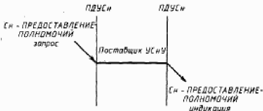
Рисунок 10 — Последовательность примитивов услуги С н -ПРЕДОСТАВЛЕНИЕ-ПОЛНОМОЧИЙ
