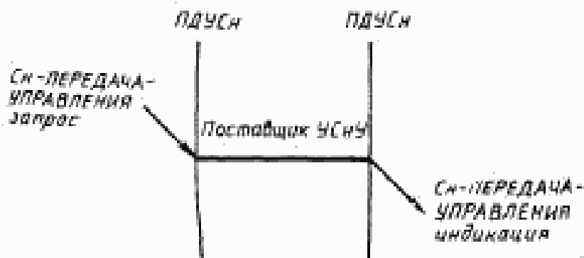
Рисунок 12 — Последовательность примитивов услуги SN-ПЕРЕДАЧА-УПРАВЛЕНИЯ
