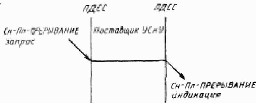
Рисунок 24 — Последовательность примитивов услуги Сл-Пл-ПРЕРЫВАНИЕ
