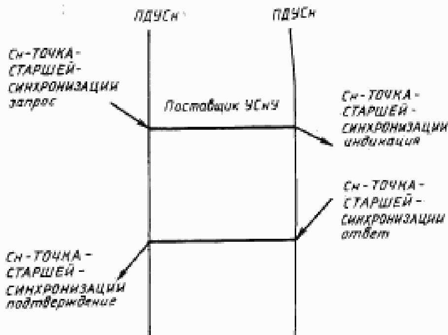
Рисунок 14 — Последовательность примитивов услуги СН-ТОЧКА-СТАРШЕЙ-СИНХРОНИЗАЦИИ
