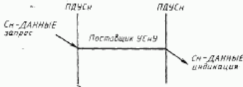
Рисунок 6 — Последовательность примитивов услуги Сн-ДААННЫЕ
