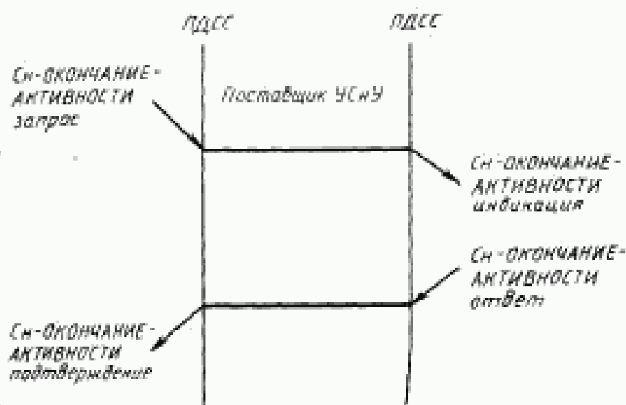
Рисунок 22 — Последовательность примитивов услуги Cn-OKONCHANIJE-AKTIVNOSTI
