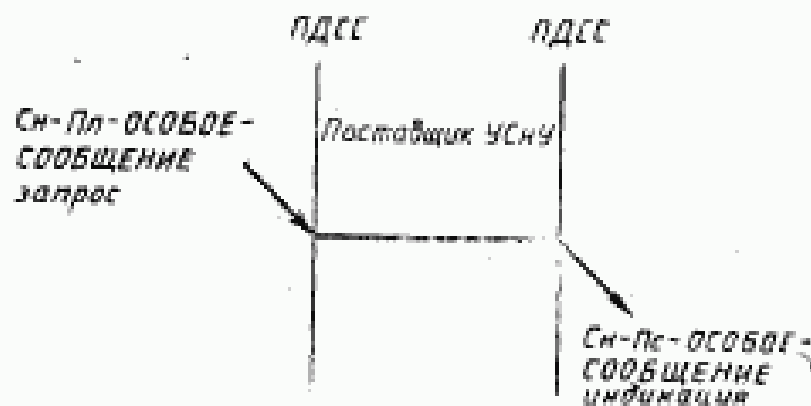
Рисунок 17 — Последовательность примитивов услуги Сл-Пл-ОСОБОЕ-СООБЩЕНИЕ
