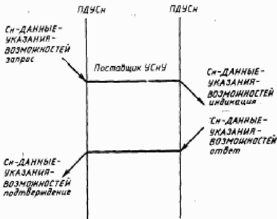
Рисунок 9 — Последовательность примитивов услуги Сл-ДААННЫЕ-УКАЗАНИЯ-ВОЗМОЖНОСТЕЙ
