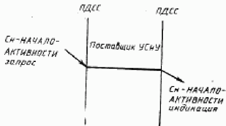
Рисунок 18 — Последовательность примитивов услуги НАЧАЛО-АКТИВНОСТИ
