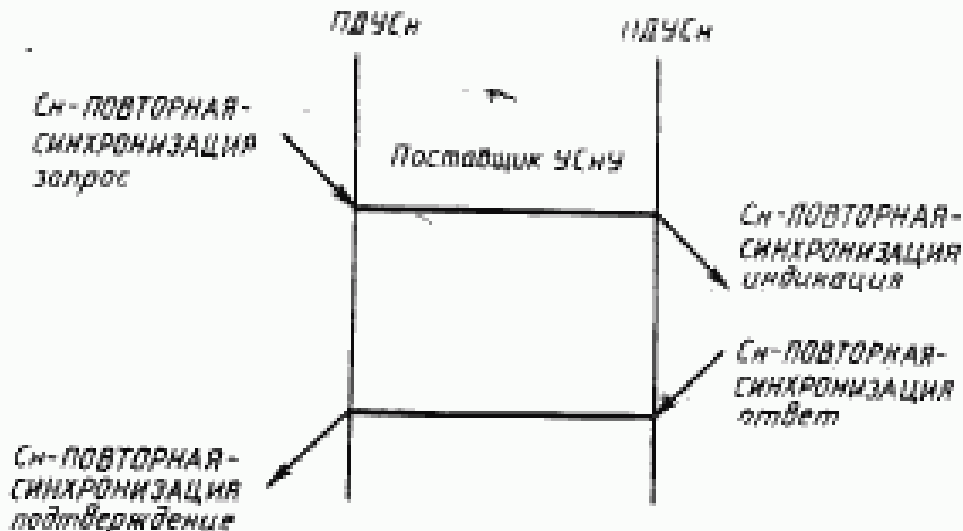
Рисунок 15 — Последовательность примитивов услуги Сн-ПОВТОРНАЯ-СИНХРОНИЗАЦИЯ
