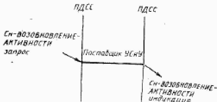
Рисунок 19 — Последовательность примитивов услуги ВОЗВООДНОВЛЕНИЕ-АКТИВНОСТИ
