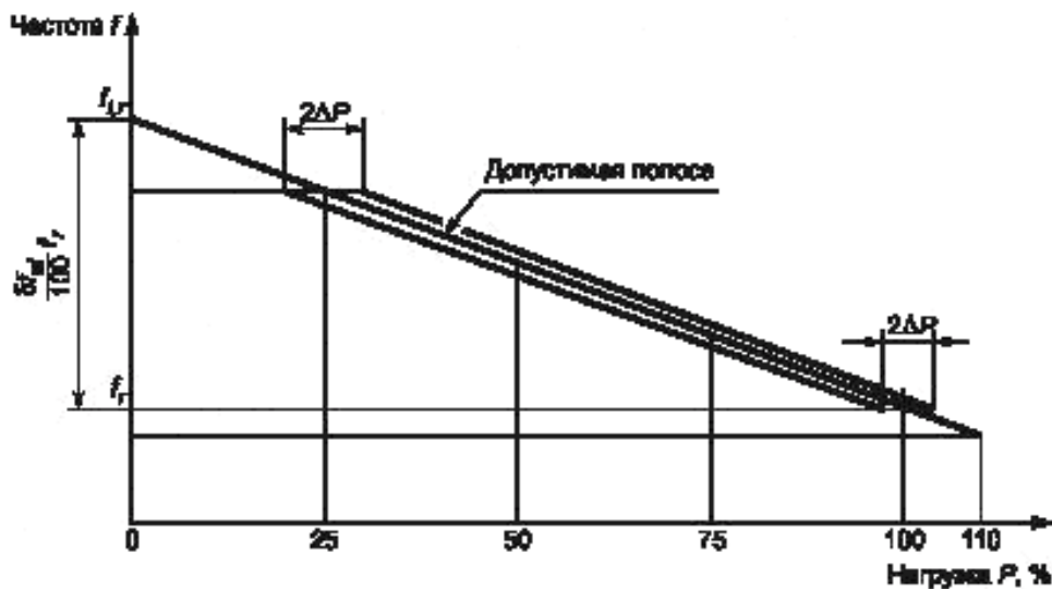
Рисунок 12 — Распределение мощности при параллельной нагрузке
