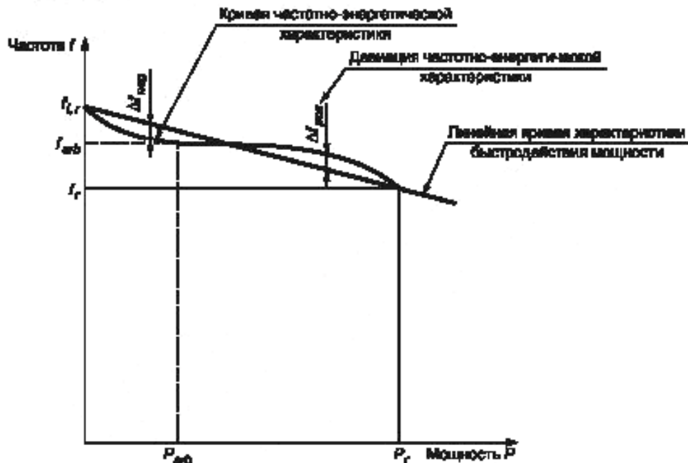
Рисунок 2 — Частотно-энергетическая характеристика отклонения от линейной кривой
