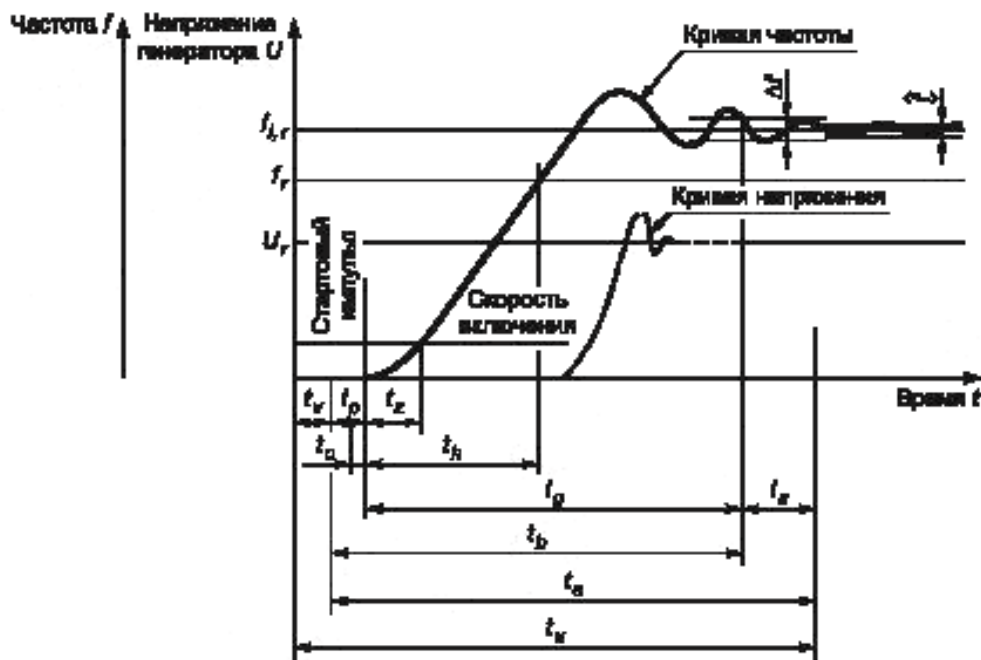
Рисунок 10 — Пусковые характеристики
