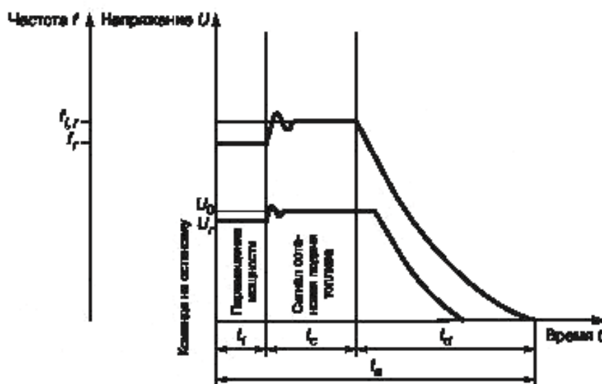
Рисунок 11 — Характеристики остановки
