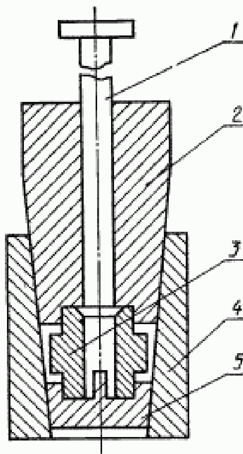
1 — пуансон; 2 — бункер; 3 — гнездо для тигля; 4 — обруч; 5 — пята
