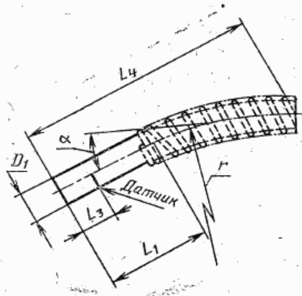
Рисунок 1 — Патрубок сливной раздаточного крана
