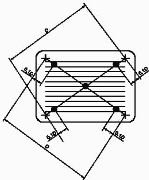
Рисунок 11 — Стандартные места измерений
