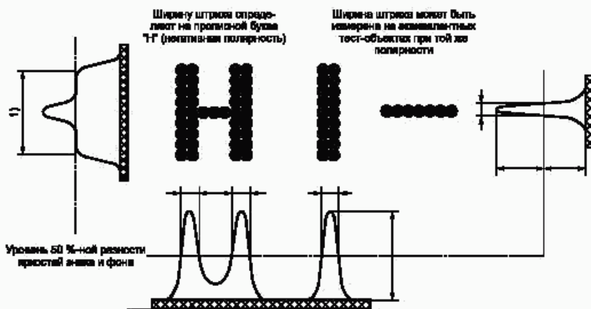
Рисунок 13 — Ширина штриха знака
