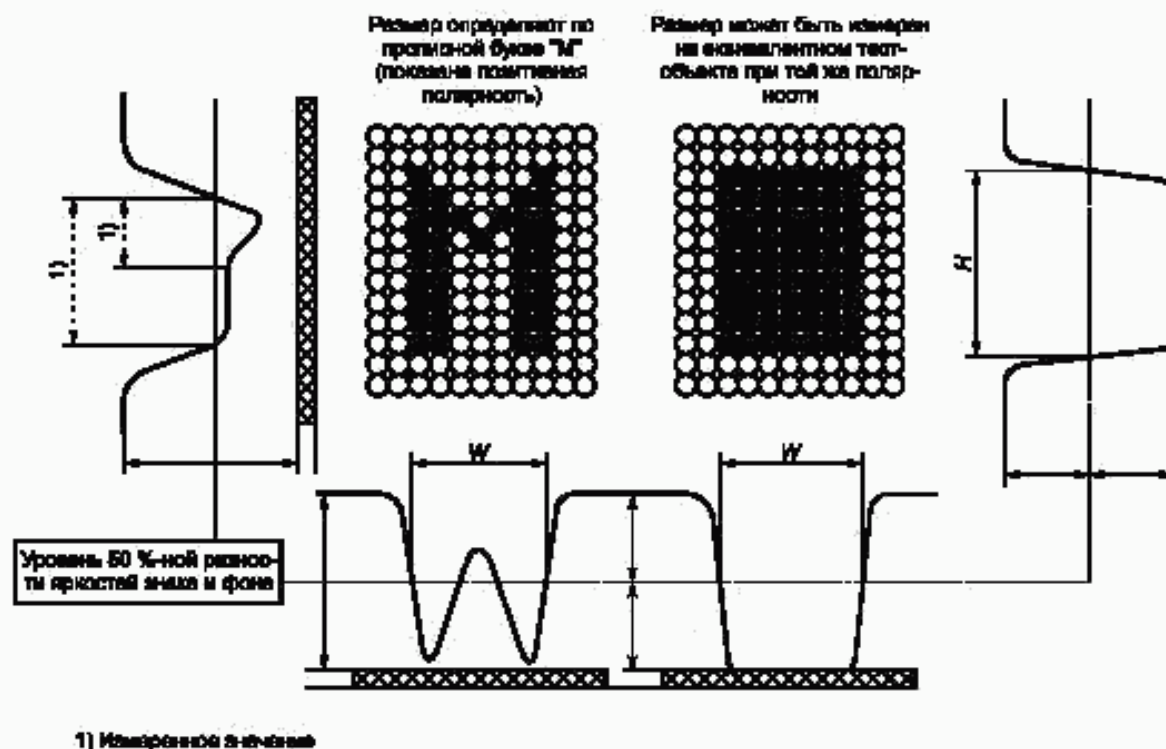
Рисунок 12 — Высота H и ширина W знака
