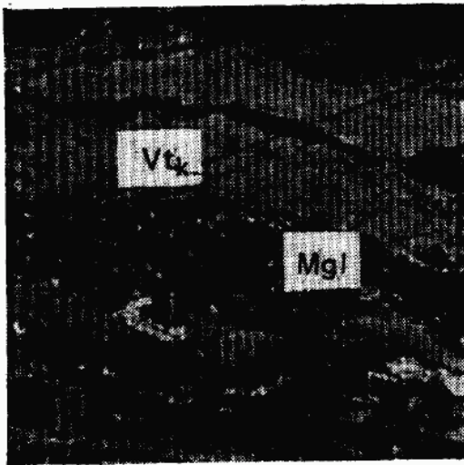
Vt_k — коллинит; M_{gl} — глинистые минералы
