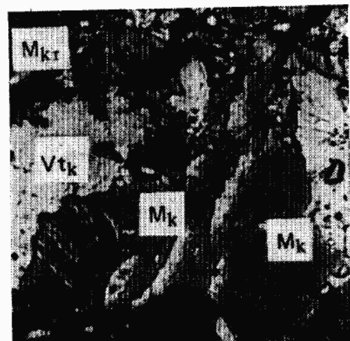
Vt_k — коллинит; M_k — карбонаты; M_{kr} — кварц
