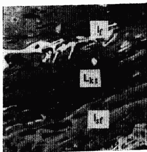
L_{kt} — кутинит; I_{sf} — семифузинит; I_f — фузинит
