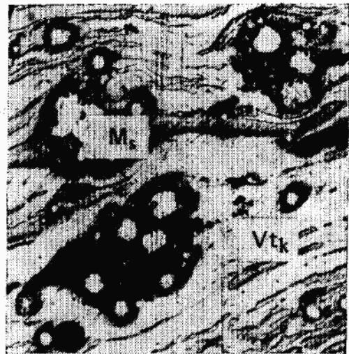
Vt_k — коллинит; M_s — сульфиды железа
