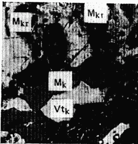
Vt_k — коллинит; M_k — карбонаты (кальцит); M_{kr} — кварц
