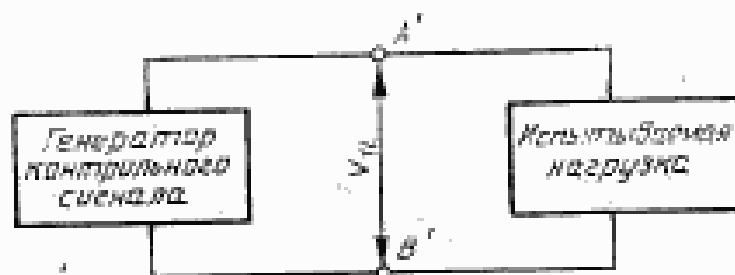
Рисунок 6 — Испытательная схема нагрузки V.11
