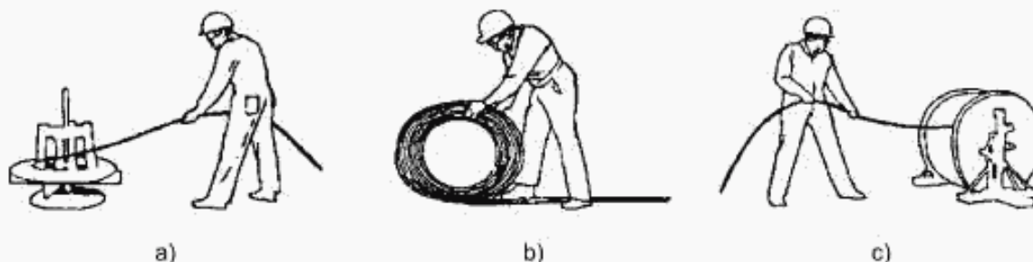
Рисунок С.1 — Разматывание
