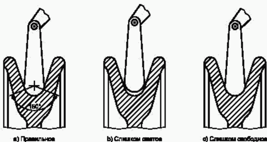
Рисунок С.4 — Проверка шкивов
