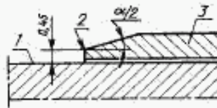
1 — поверхность стебля; 2 — измерительная кромка; 3 — барабан
